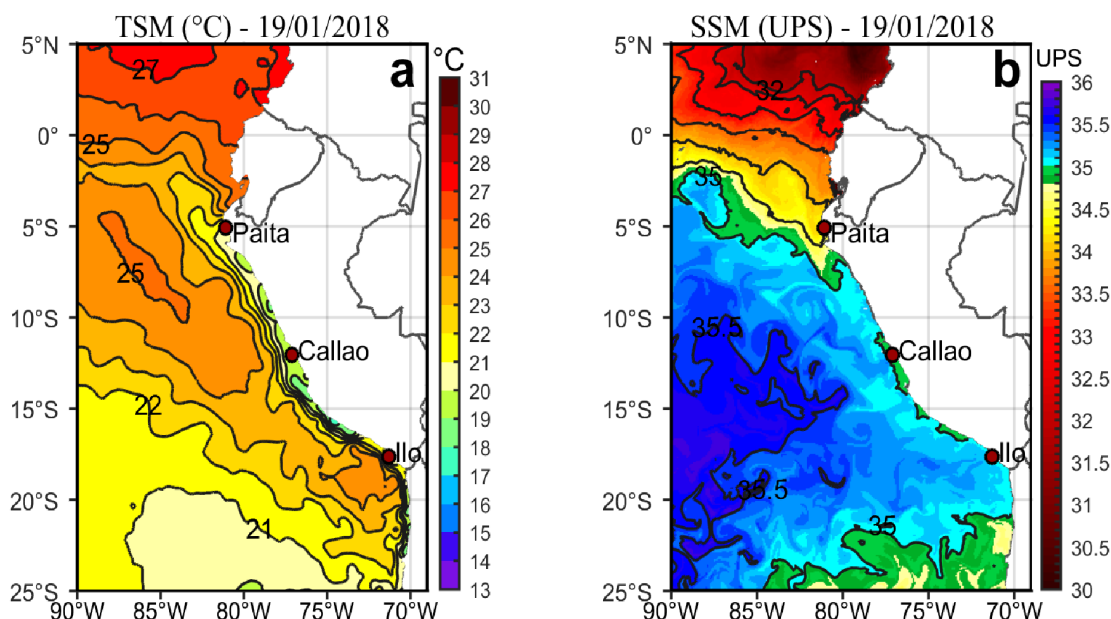
Figura 2. a) Temperatura superficial del mar ( ^{\circ}\text{C} ) y b) Salinidad superficial del mar (UPS) para el 19 de enero de 2018. Datos: OSTIA-UKMO-L4-GLOB-v2.0 (UK Met Office, 2012; Donlon et al, 2012) disponible en https://podaac.jpl.nasa.gov/dataset/OSTIA-UKMO-L4-GLOB-v2.0 para (a) y Hybrid Coordinate Ocean Model (HYCOM; Halliwell et al., 1998; 2000; Bleck, 2001) para (b). Procesamiento: LHF/AFIOF/DGIOCC/IMARPE.
