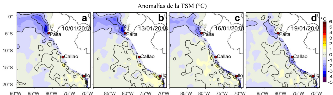
Figura 3. Anomalías de la Temperatura Superficial del Mar ( ^{\circ}\text{C} ) para los días: a) 10, b) 13, c) 16 y d) 19 de enero de 2018. Las anomalías se calcularon respecto de la climatología para el periodo 2007-2016. Datos: OSTIA-UKMO-L4-GLOB-v2.0 (UK Met Office, 2012; Donlon et al, 2012). Procesamiento: LHF/AFIOF/DGIOCC/IMARPE.
