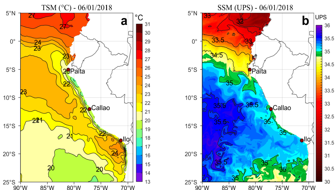
Figura 2. a) Temperatura superficial del mar (°C) y b) Salinidad superficial del mar (UPS) para el 06 de enero. Datos: OSTIA-UKMO-L4-GLOB-v2.0 (UK Met Office, 2012; Donlon et al, 2012) disponible en https://podaac.jpl.nasa.gov/dataset/OSTIA-UKMO-L4-GLOB-v2.0 para (a) y Hybrid Coordinate Ocean Model (HYCOM; Halliwell et al., 1998; 2000; Bleck, 2001) para (b). Procesamiento: LHF/AFIOF/DGIOCC/IMARPE.
