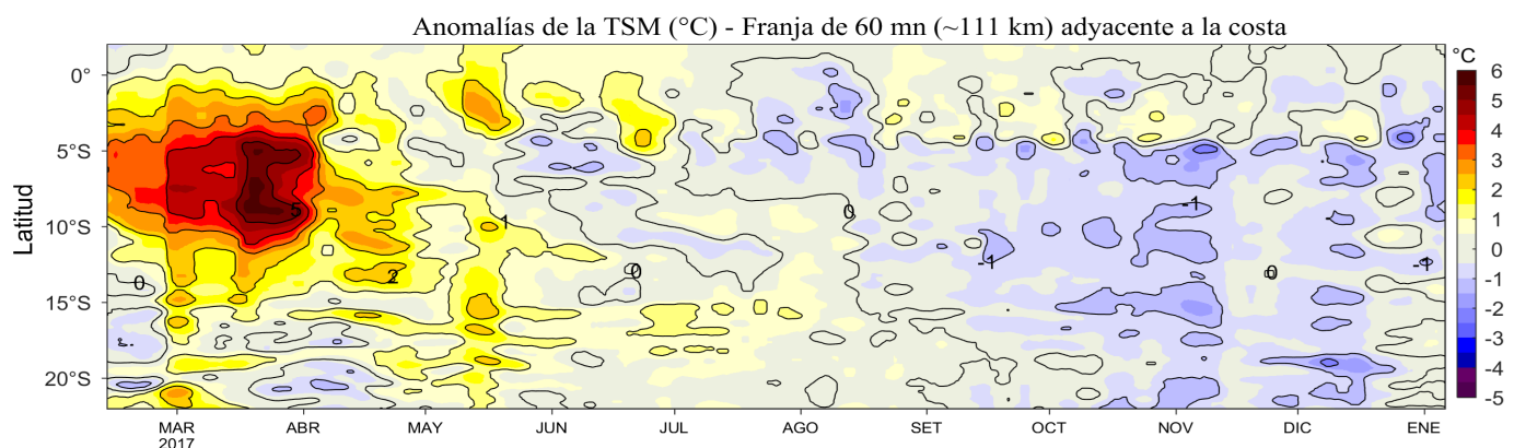
Figura 4. Variación promedio de las anomalías de la temperatura superficial del mar (°C) para una franja de 60 mn (~111 km) adyacente al litoral peruano para los últimos doce meses al 06 de diciembre de 2017. Datos: OSTIA-UKMO-L4-GLOB-v2.0 (UK Met. Office, 2012; Donlon et al, 2012) disponible en https://podaac.jpl.nasa.gov/dataset/OSTIA-UKMO-L4-GLOB-v2.0 . Las anomalías se calcularon con respecto al periodo 2007-2016. Procesamiento: LHF/AFIOF/DGIOCC/IMARPE.
