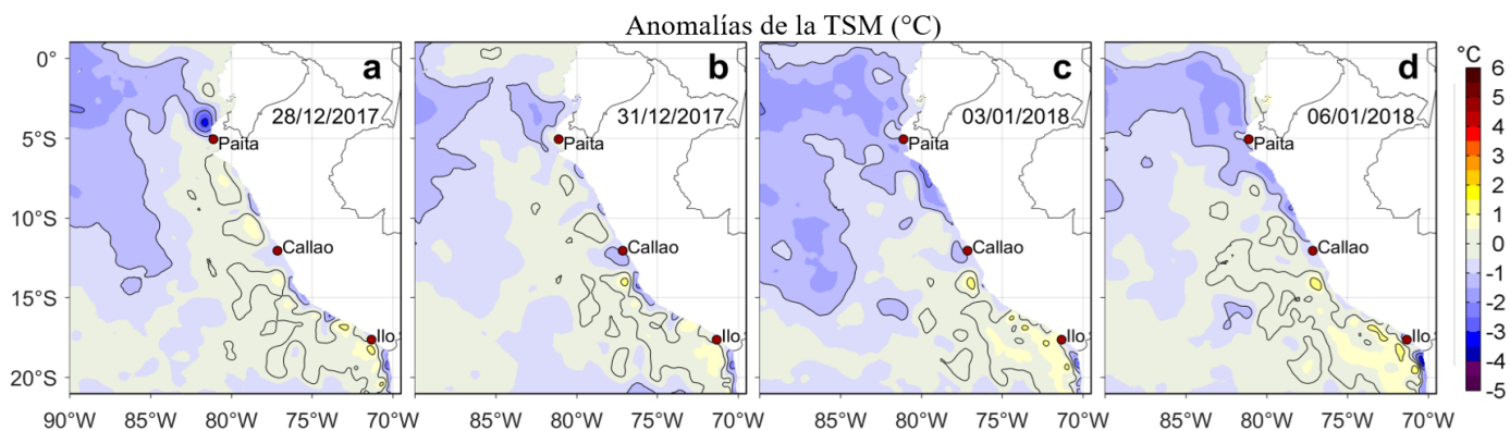
Figura 3. Anomalías de la Temperatura Superficial del Mar (°C) para los días: a) 28 y b) 31 de diciembre de 2017, y c) 03 y d) 06 de enero de 2018. Las anomalías se calcularon respecto de la climatología para el periodo 2007-2016. Datos: OSTIA-UKMO-L4-GLOB-v2.0 (UK Met Office, 2012; Donlon et al, 2012). Procesamiento: LHF/AFIOF/DGIOCC/IMARPE.
