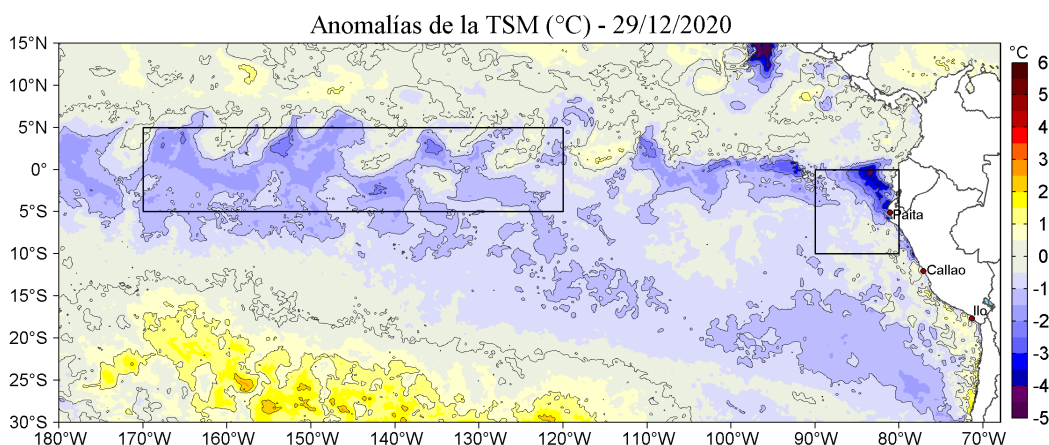
Figura 1. Anomalías de la temperatura superficial del mar (TSM, °C) en el océano Pacífico tropical. Las regiones Niño 3.4 (5 °N- 5 °S, 170 °W - 120 °W) y Niño 1+2 (0 - 10 °S, 90 °W - 80 °W) en los sectores central y oriental del océano, respectivamente, están delimitadas con una línea de color negro. Climatología: 2007-2016. Datos: OSTIA-UKMO-L4-GLOB-v2.0 (UK Met Office, 2012; Donlon et al, 2012) disponible en https://podaac.jpl.nasa.gov/dataset/OSTIA-UKMO-L4-GLOB-v2.0 . Procesamiento: LHFM/AFIOF/DGIOCC.
