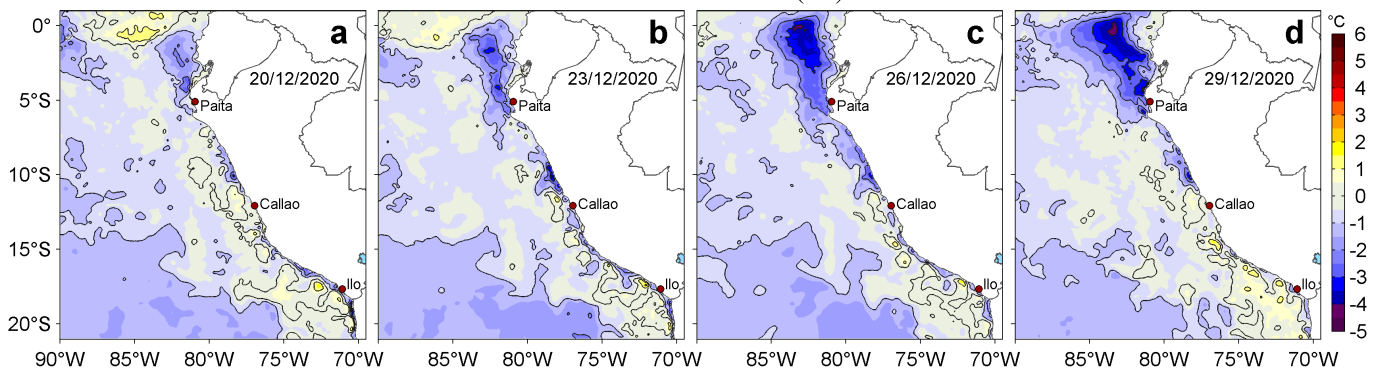
Figura 3. Anomalías de la temperatura superficial del mar (TSM, °C) para los días: a) 20, b) 23, c) 26 y d) 29 de diciembre de 2020. Las anomalías se calcularon respecto de la climatología para el periodo 2007-2016. Datos: OSTIA-UKMO-L4-GLOB-v2.0 (UK Met Office, 2012; Donlon et al, 2012). Procesamiento: LHF/AFIOF/DGIOCC.
