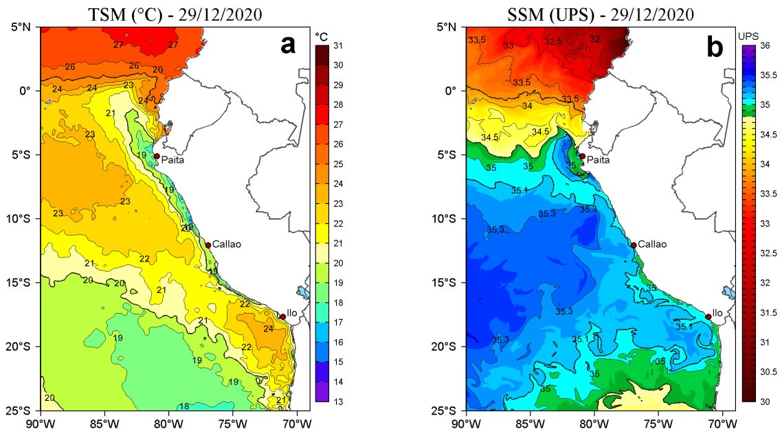
Figura 2. a) Temperatura superficial del mar (TSM, °C) y b) Salinidad superficial del mar (SSM, UPS), para el 29 de diciembre de 2020. Datos: OSTIA-UKMO-L4-GLOB-v2.0 (UK Met Office, 2012; Donlon et al, 2012) disponible en https://podaac.jpl.nasa.gov/dataset/OSTIA-UKMO-L4-GLOB-v2.0 para (a) y Hybrid Coordinate Ocean Model v. GOF3.1 (HYCOM; Halliwell et al., 1998; 2000; Bleck, 2001) para (b). Procesamiento: LHF/AFIOF/DGIOCC.
