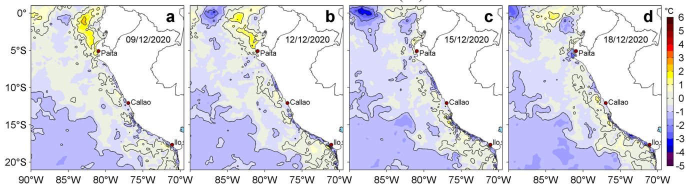
Figura 3. Anomalías de la temperatura superficial del mar (TSM, °C) para los días: a) 09, b) 12, c) 15 y d) 18 de diciembre de 2020. Las anomalías se calcularon respecto de la climatología para el periodo 2007-2016. Datos: OSTIA-UKMO-L4-GLOB-v2.0 (UK Met Office, 2012; Donlon et al, 2012). Procesamiento: LHFMAFIOF/DGIOCC.
