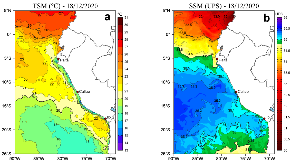
Figura 2. a) Temperatura superficial del mar (TSM, °C) y b) Salinidad superficial del mar (SSM, UPS), para el 18 de diciembre de 2020. Datos: OSTIA-UKMO-L4-GLOB-v2.0 (UK Met Office, 2012; Donlon et al, 2012) disponible en https://podaac.jpl.nasa.gov/dataset/OSTIA-UKMO-L4-GLOB-v2.0 para (a) y Hybrid Coordinate Ocean Model v. GOFS 3.1 (HYCOM; Halliwell et al., 1998; 2000; Bleck, 2001) para (b). Procesamiento: LHFMAFIOF/DGIOCC.
