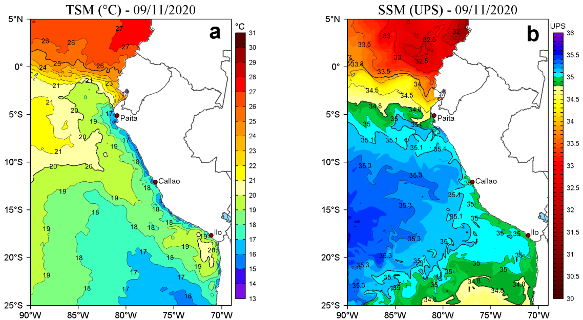
Figura 2. a) Temperatura superficial del mar (TSM, °C) y b) Salinidad superficial del mar (SSM, UPS), para el 09 de noviembre de 2020. Datos: OSTIA-UKMO-L4-GLOB-v2.0 (UK Met Office, 2012; Donlon et al, 2012) disponible en https://podaac.jpl.nasa.gov/dataset/OSTIA-UKMO-L4-GLOB-v2.0 para (a) y Hybrid Coordinate Ocean Model v. GOFS 3.1 (HYCOM; Halliwell et al., 1998; 2000; Bleck, 2001) para (b). Procesamiento: LHFMAF/AFIOF/DGIOCC.
