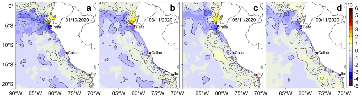
Figura 3. Anomalías de la temperatura superficial del mar (TSM, °C) para los días: a) 31 de octubre, b) 03, c) 06 y d) 09 de noviembre de 2020. Las anomalías se calcularon respecto de la climatología para el periodo 2007-2016. Datos: OSTIA-UKMO-L4-GLOB-v2.0 (UK Met Office, 2012; Donlon et al, 2012). Procesamiento: LHFMAF/AFIOF/DGIOCC.
