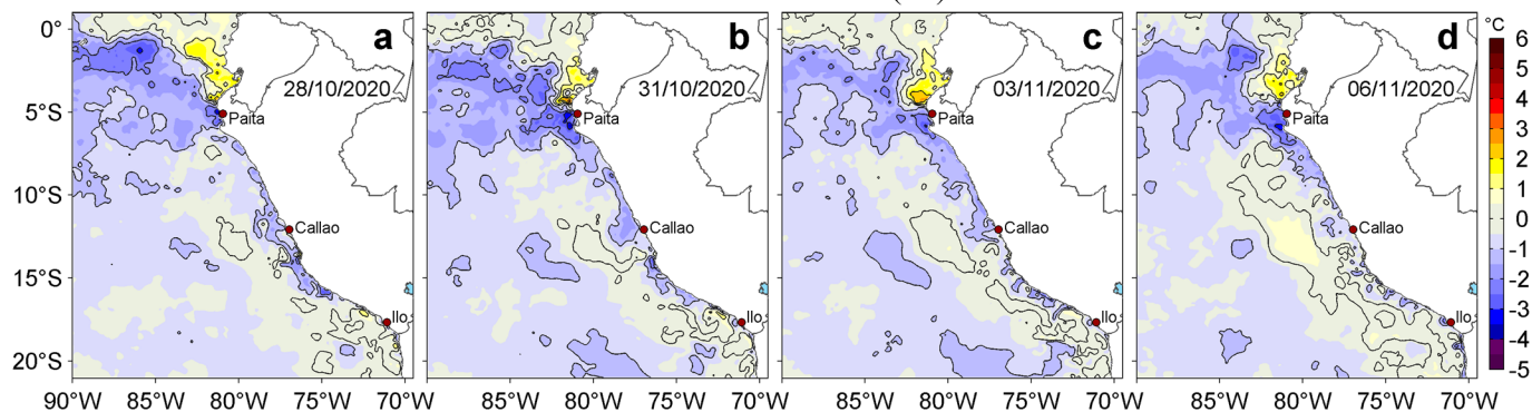
Figura 3. Anomalías de la temperatura superficial del mar (TSM, °C) para los días: a) 28 y b) 31 de octubre, c) 03 y d) 06 de noviembre de 2020. Las anomalías se calcularon respecto de la climatología para el periodo 2007-2016. Datos: OSTIA-UKMO-L4-GLOB-v2.0 (UK Met Office, 2012; Donlon et al, 2012). Procesamiento: LHF/AFIOF/DGIOCC.
