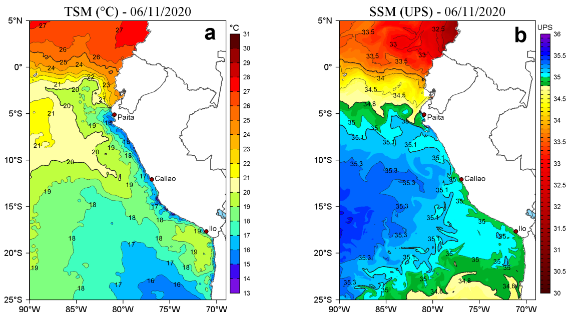
Figura 2. a) Temperatura superficial del mar (TSM, °C) y b) Salinidad superficial del mar (SSM, UPS), para el 06 de noviembre de 2020. Datos: OSTIA-UKMO-L4-GLOB-v2.0 (UK Met Office, 2012; Donlon et al, 2012) disponible en https://podaac.jpl.nasa.gov/dataset/OSTIA-UKMO-L4-GLOB-v2.0 para (a) y Hybrid Coordinate Ocean Model v. GOFS 3.1 (HYCOM; Halliwell et al., 1998; 2000; Bleck, 2001) para (b). Procesamiento: LHF/AFIOF/DGIOCC.
