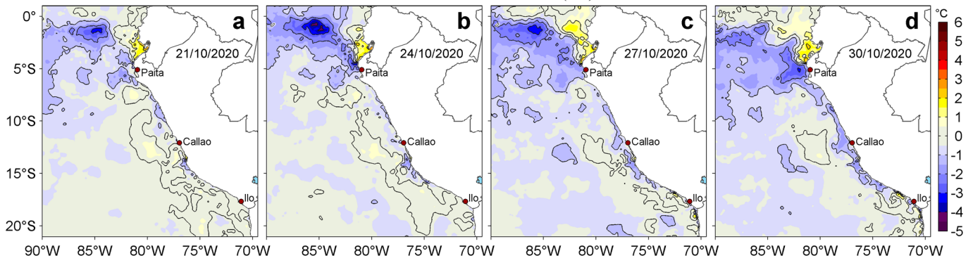
Figura 3. Anomalías de la temperatura superficial del mar (TSM, °C) para los días: a) 21, b) 24, c) 27 y d) 30 de octubre de 2020. Las anomalías se calcularon respecto de la climatología para el periodo 2007-2016. Datos: OSTIA-UKMO-L4-GLOB-v2.0 (UK Met Office, 2012; Donlon et al, 2012). Procesamiento: LHFm/AFIOF/DGIOCC.
