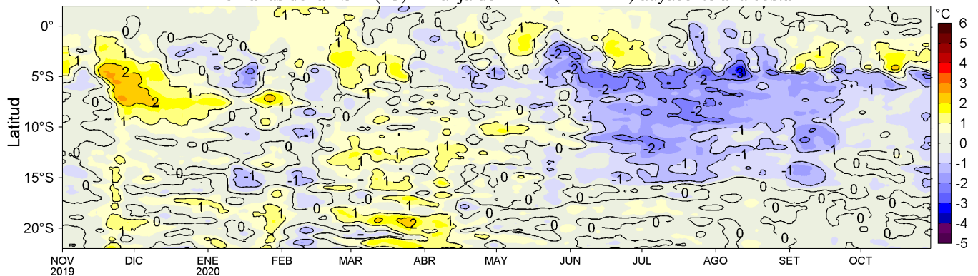
Figura 4. Variación promedio de las anomalías de la temperatura superficial del mar (TSM, °C) para una franja de 60 mn (~111 km) adyacente al litoral peruano para los últimos doce meses al 30 de octubre de 2020. Datos: OSTIA-UKMO-L4-GLOB-v2.0 (UK Met. Office, 2012; Donlon et al, 2012) disponible en https://podaac.jpl.nasa.gov/dataset/OSTIA-UKMO-L4-GLOB-v2.0 . Las anomalías se calcularon con respecto al periodo 2007-2016. Procesamiento: LHFm/AFIOF/DGIOCC.
