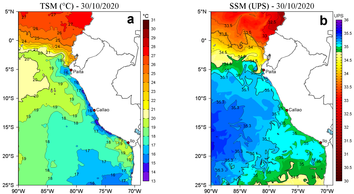
Figura 2. a) Temperatura superficial del mar (TSM, °C) y b) Salinidad superficial del mar (SSM, UPS), para el 30 de octubre de 2020. Datos: OSTIA-UKMO-L4-GLOB-v2.0 (UK Met Office, 2012; Donlon et al, 2012) disponible en https://podaac.jpl.nasa.gov/dataset/OSTIA-UKMO-L4-GLOB-v2.0 para (a) y Hybrid Coordinate Ocean Model v. GOFS 3.1 (HYCOM; Halliwell et al., 1998; 2000; Bleck, 2001) para (b). Procesamiento: LHFm/AFIOF/DGIOCC.
