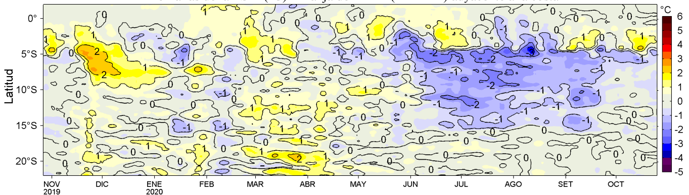
Figura 4. Variación promedio de las anomalías de la temperatura superficial del mar (TSM, °C) para una franja de 60 m.n. (~111 km) adyacente al litoral peruano para los últimos doce meses al 25 de octubre de 2020. Datos: OSTIA-UKMO-L4-GLOB-v2.0 (UK Met. Office, 2012; Donlon et al, 2012) disponible en https://podaac.jpl.nasa.gov/dataset/OSTIA-UKMO-L4-GLOB-v2.0 . Las anomalías se calcularon con respecto al periodo 2007-2016. Procesamiento: LHF/AFIOF/DGIOCC.
