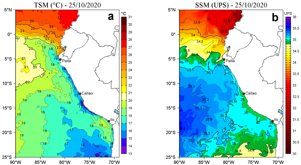
Figura 2. a) Temperatura superficial del mar (TSM, °C) y b) Salinidad superficial del mar (SSM, UPS), para el 25 de octubre de 2020. Datos: OSTIA-UKMO-L4-GLOB-v2.0 (UK Met Office, 2012; Donlon et al, 2012) disponible en https://podaac.jpl.nasa.gov/dataset/OSTIA-UKMO-L4-GLOB-v2.0 para (a) y Hybrid Coordinate Ocean Model v. GOF3 3.1 (HYCOM; Halliwell et al., 1998; 2000; Bleck, 2001) para (b). Procesamiento: LHF/AFIOF/DGIOCC.
