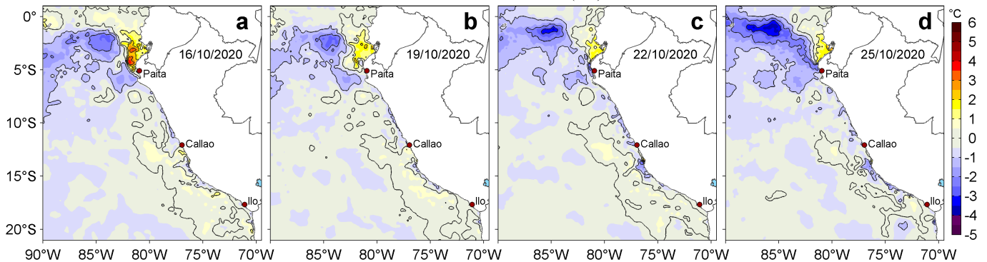
Figura 3. Anomalías de la temperatura superficial del mar (TSM, °C) para los días: a) 16, b) 19, c) 22 y d) 25 de octubre de 2020. Las anomalías se calcularon respecto de la climatología para el periodo 2007-2016. Datos: OSTIA-UKMO-L4-GLOB-v2.0 (UK Met Office, 2012; Donlon et al, 2012). Procesamiento: LHF/AFIOF/DGIOCC.
