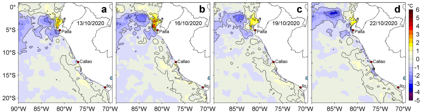
Figura 3. Anomalías de la temperatura superficial del mar (TSM, °C) para los días: a) 13, b) 16, c) 19 y d) 22 de octubre de 2020. Las anomalías se calcularon respecto de la climatología para el periodo 2007-2016. Datos: OSTIA-UKMO-L4-GLOB-v2.0 (UK Met Office, 2012; Donlon et al, 2012). Procesamiento: LHF/AFIOF/DGIOCC.
