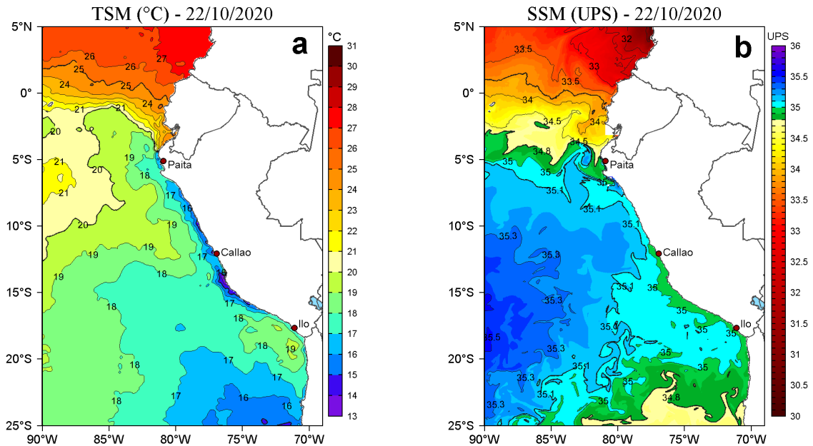
Figura 2. a) Temperatura superficial del mar (TSM, °C) y b) Salinidad superficial del mar (SSM, UPS), para el 22 de octubre de 2020. Datos: OSTIA-UKMO-L4-GLOB-v2.0 (UK Met Office, 2012; Donlon et al, 2012) disponible en https://podaac.jpl.nasa.gov/dataset/OSTIA-UKMO-L4-GLOB-v2.0 para (a) y Hybrid Coordinate Ocean Model v. GOFS 3.1 (HYCOM; Halliwell et al., 1998; 2000; Bleck, 2001) para (b). Procesamiento: LHF/AFIOF/DGIOCC.
