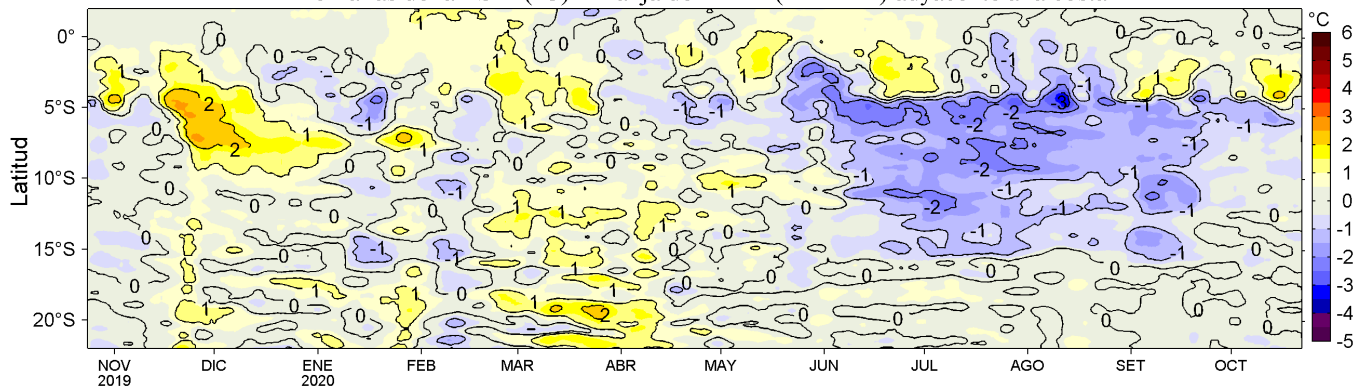
Figura 4. Variación promedio de las anomalías de la temperatura superficial del mar (TSM, °C) para una franja de 60 mn (~111 km) adyacente al litoral peruano para los últimos doce meses al 22 de octubre de 2020. Datos: OSTIA-UKMO-L4-GLOB-v2.0 (UK Met. Office, 2012; Donlon et al, 2012) disponible en https://podaac.jpl.nasa.gov/dataset/OSTIA-UKMO-L4-GLOB-v2.0 . Las anomalías se calcularon respecto al periodo 2007-2016. Procesamiento: LHF/AFIOF/DGIOCC.
