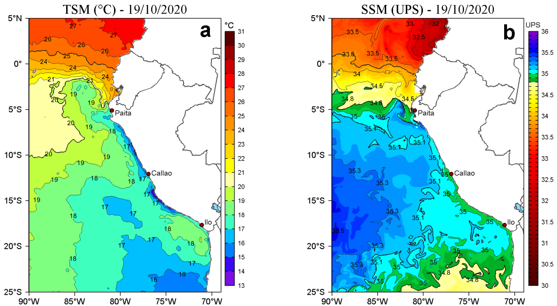
Figura 2. a) Temperatura superficial del mar (TSM, °C) y b) Salinidad superficial del mar (SSM, UPS), para el 19 de octubre de 2020. Datos: OSTIA-UKMO-L4-GLOB-v2.0 (UK Met Office, 2012; Donlon et al, 2012) disponible en https://podaac.jpl.nasa.gov/dataset/OSTIA-UKMO-L4-GLOB-v2.0 para (a) y Hybrid Coordinate Ocean Model v. GOFS 3.1 (HYCOM; Halliwell et al., 1998; 2000; Bleck, 2001) para (b). Procesamiento: LHF/AFIOF/DGIOCC.
