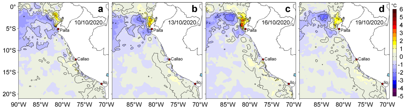
Figura 3. Anomalías de la temperatura superficial del mar (TSM, °C) para los días: a) 10, b) 13, c) 16 y d) 19 de octubre de 2020. Las anomalías se calcularon respecto de la climatología para el periodo 2007-2016. Datos: OSTIA-UKMO-L4-GLOB-v2.0 (UK Met Office, 2012; Donlon et al, 2012). Procesamiento: LHF/AFIOF/DGIOCC.
