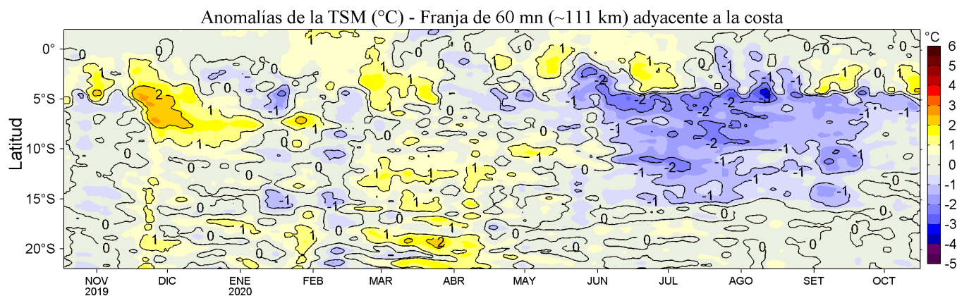
Figura 4. Variación promedio de las anomalías de la temperatura superficial del mar (TSM, °C) para una franja de 60 mn (~111 km) adyacente al litoral peruano para los últimos doce meses al 16 de octubre de 2020. Datos: OSTIA-UKMO-L4-GLOB-v2.0 (UK Met. Office, 2012; Donlon et al, 2012) disponible en https://podaac.jpl.nasa.gov/dataset/OSTIA-UKMO-L4-GLOB-v2.0 . Las anomalías se calcularon con respecto al periodo 2007-2016. Procesamiento: LHF/AFIOF/DGIOCC.
