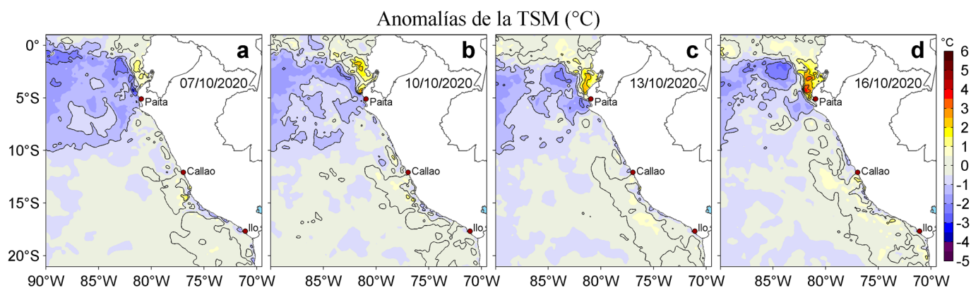
Figura 3. Anomalías de la temperatura superficial del mar (TSM, °C) para los días: a) 07, b) 10, c) 13 y d) 16 de octubre de 2020. Las anomalías se calcularon respecto de la climatología para el periodo 2007-2016. Datos: OSTIA-UKMO-L4-GLOB-v2.0 (UK Met Office, 2012; Donlon et al, 2012). Procesamiento: LHF/AFIOF/DGIOCC.
