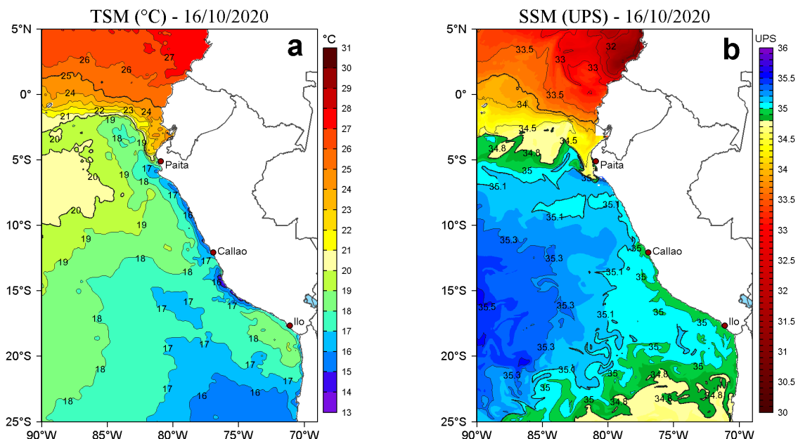
Figura 2. a) Temperatura superficial del mar (TSM, °C) y b) Salinidad superficial del mar (SSM, UPS), para el 16 de octubre de 2020. Datos: OSTIA-UKMO-L4-GLOB-v2.0 (UK Met Office, 2012; Donlon et al, 2012) disponible en https://podaac.jpl.nasa.gov/dataset/OSTIA-UKMO-L4-GLOB-v2.0 para (a) y Hybrid Coordinate Ocean Model v. GOFS 3.1 (HYCOM; Halliwell et al., 1998; 2000; Bleck, 2001) para (b). Procesamiento: LHF/AFIOF/DGIOCC.
