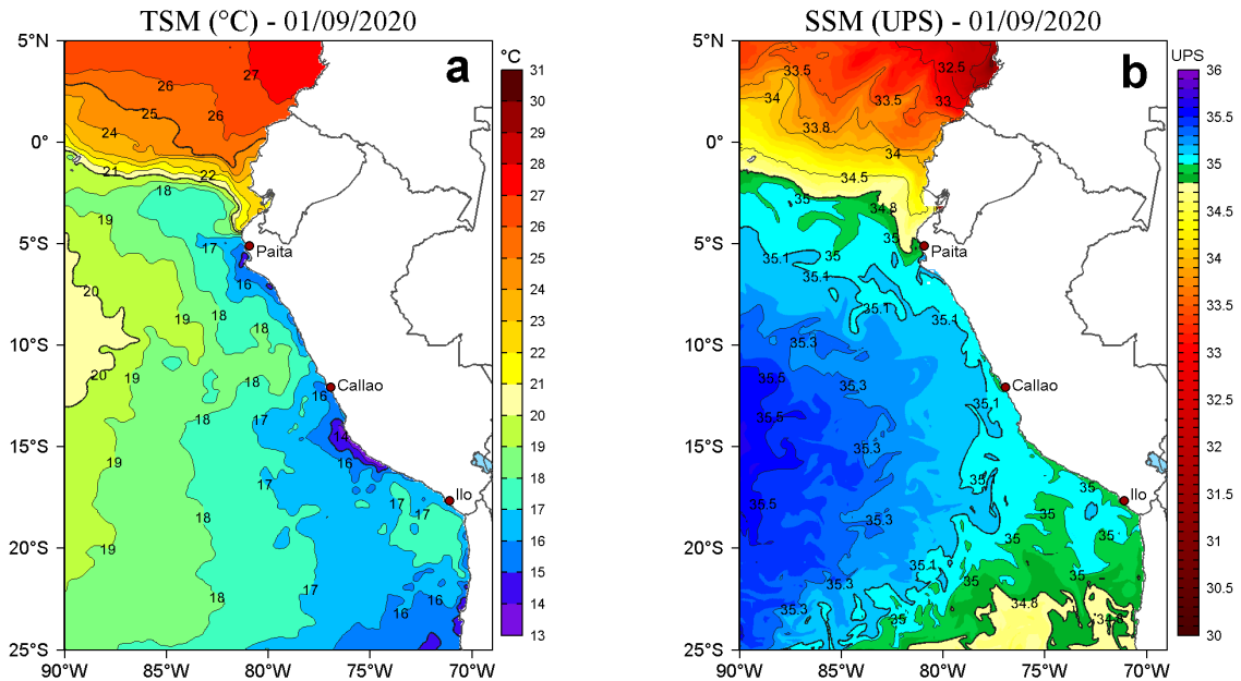
Figura 2. a) Temperatura superficial del mar (TSM, °C) y b) Salinidad superficial del mar (SSM, UPS), para el 01 de setiembre de 2020. Datos: OSTIA-UKMO-L4-GLOB-v2.0 (UK Met Office, 2012; Donlon et al, 2012) disponible en https://podaac.jpl.nasa.gov/dataset/OSTIA-UKMO-L4-GLOB-v2.0 para (a) y Hybrid Coordinate Ocean Model v. GOFS 3.1 (HYCOM; Halliwell et al., 1998; 2000; Bleck, 2001) para (b). Procesamiento: LHFMA/AFIOF/DGIOCC.
