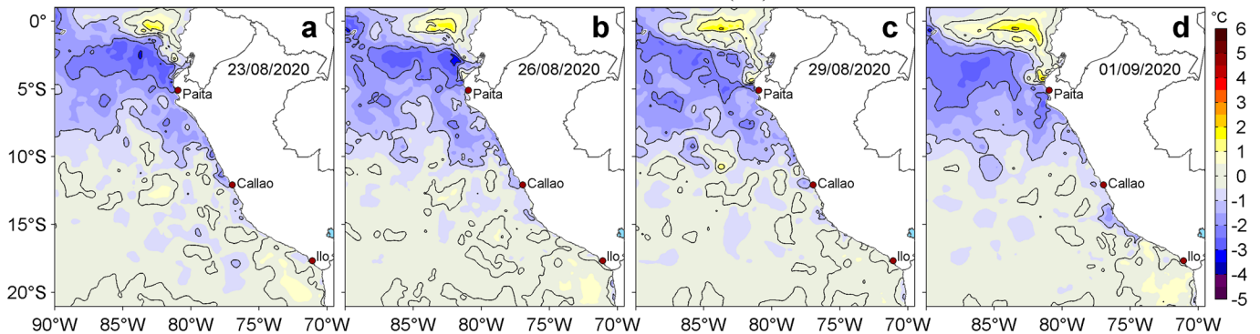
Figura 3. Anomalías de la temperatura superficial del mar (TSM, °C) para los días: a) 23, b) 26 y c) 29 de agosto, d) 01 de setiembre de 2020. Las anomalías se calcularon respecto de la climatología para el periodo 2007-2016. Datos: OSTIA-UKMO-L4-GLOB-v2.0 (UK Met Office, 2012; Donlon et al, 2012). Procesamiento: LHFMA/AFIOF/DGIOCC.
