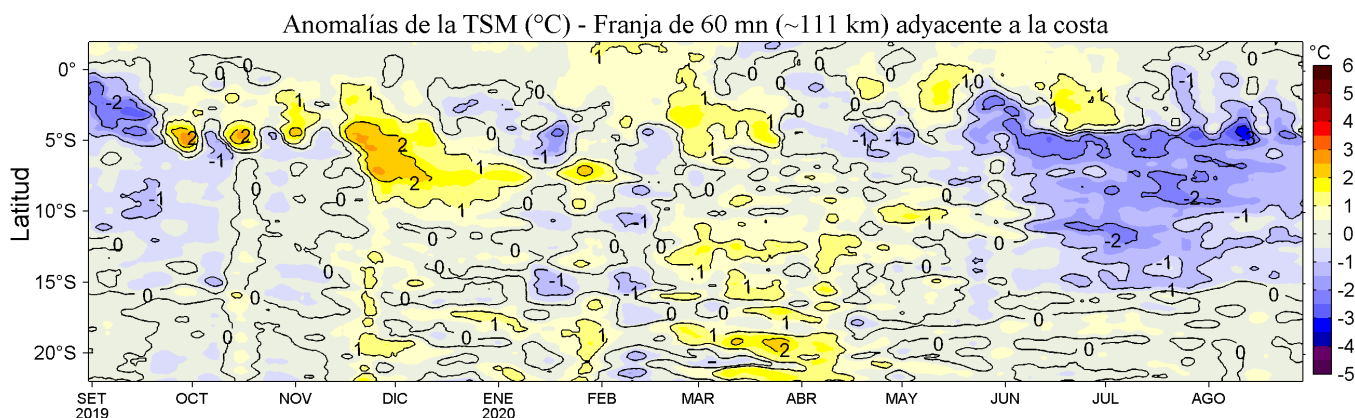
Figura 4. Variación promedio de las anomalías de la temperatura superficial del mar (TSM, °C) para una franja de 60 mn (~111 km) adyacente al litoral peruano para los últimos doce meses al 29 de agosto de 2020. Datos: OSTIA-UKMO-L4-GLOB-v2.0 (UK Met. Office, 2012; Donlon et al, 2012) disponible en https://podaac.jpl.nasa.gov/dataset/OSTIA-UKMO-L4-GLOB-v2.0 . Las anomalías se calcularon con respecto al periodo 2007-2016. Procesamiento: LHF/AFIOF/DGIOCC.
