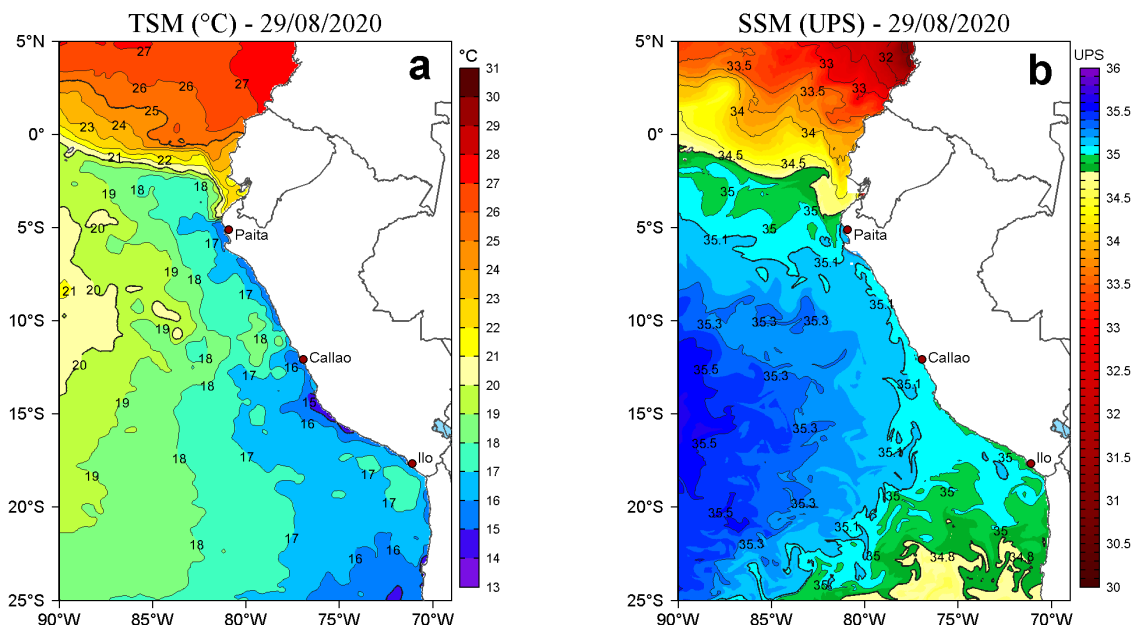
Figura 2. a) Temperatura superficial del mar (TSM, °C) y b) Salinidad superficial del mar (SSM, UPS), para el 29 de agosto de 2020. Datos: OSTIA-UKMO-L4-GLOB-v2.0 (UK Met Office, 2012; Donlon et al, 2012) disponible en https://podaac.jpl.nasa.gov/dataset/OSTIA-UKMO-L4-GLOB-v2.0 para (a) y Hybrid Coordinate Ocean Model v. GOFS 3.1 (HYCOM; Halliwell et al., 1998; 2000; Bleck, 2001) para (b). Procesamiento: LHF/AFIOF/DGIOCC.
