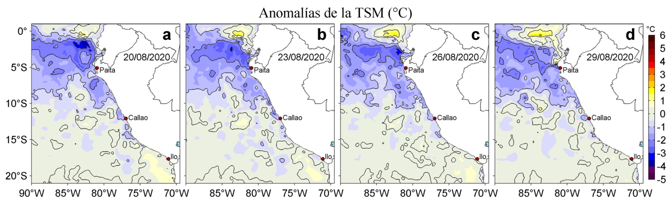
Figura 3. Anomalías de la temperatura superficial del mar (TSM, °C) para los días: a) 20, b) 23, c) 26 y d) 29 de agosto de 2020. Las anomalías se calcularon respecto de la climatología para el periodo 2007-2016. Datos: OSTIA-UKMO-L4-GLOB-v2.0 (UK Met Office, 2012; Donlon et al, 2012). Procesamiento: LHF/AFIOF/DGIOCC.
