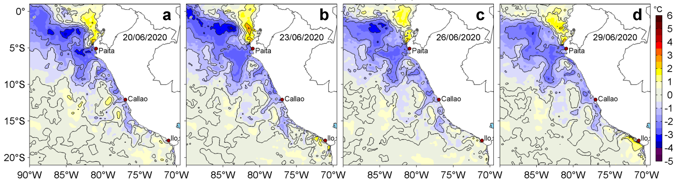
Figura 3. Anomalías de la temperatura superficial del mar (TSM, °C) para los días: a) 20, b) 23, c) 26 y d) 29 de junio de 2020. Las anomalías se calcularon respecto de la climatología para el periodo 2007-2016. Datos: OSTIA-UKMO-L4-GLOB-v2.0 (UK Met Office, 2012; Donlon et al, 2012). Procesamiento: LHF/AFIOF/DGIOCC/IMARPE.
