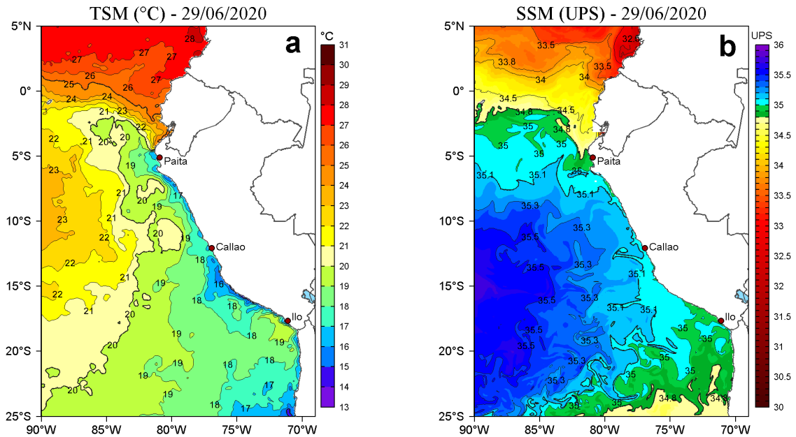
Figura 2. a) Temperatura superficial del mar (TSM, °C) y b) Salinidad superficial del mar (SSM, UPS), para el 29 de junio de 2020. Datos: OSTIA-UKMO-L4-GLOB-v2.0 (UK Met Office, 2012; Donlon et al, 2012) disponible en https://podaac.jpl.nasa.gov/dataset/OSTIA-UKMO-L4-GLOB-v2.0 para (a) y Hybrid Coordinate Ocean Model v. GOF3 3.1 (HYCOM; Halliwell et al., 1998; 2000; Bleck, 2001) para (b). Procesamiento: LHF/AFIOF/DGIOCC/IMARPE.
