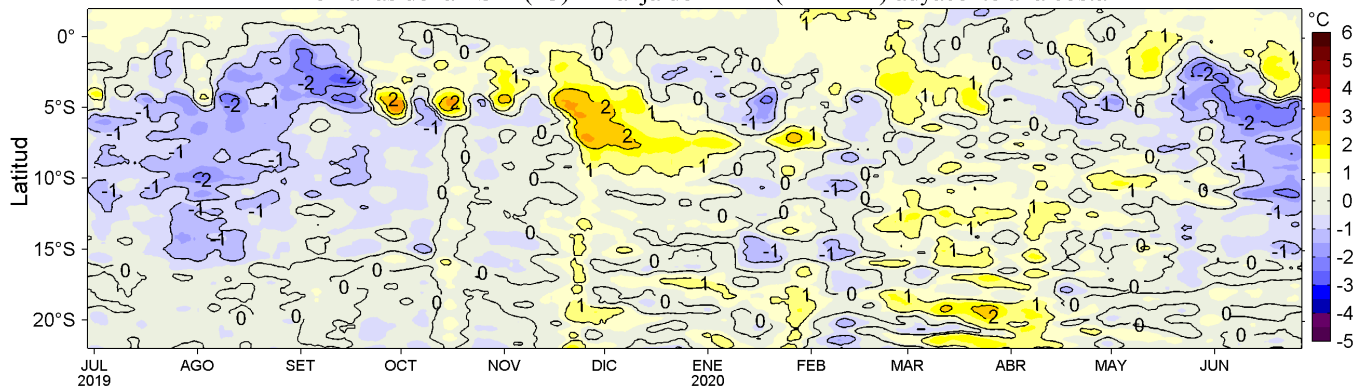
Figura 4. Variación promedio de las anomalías de la temperatura superficial del mar (TSM, °C) para una franja de 60 mn (~111 km) adyacente al litoral peruano para los últimos doce meses al 27 de junio de 2020. Datos: OSTIA-UKMO-L4-GLOB-v2.0 (UK Met. Office, 2012; Donlon et al, 2012) disponible en https://podaac.jpl.nasa.gov/dataset/OSTIA-UKMO-L4-GLOB-v2.0 . Las anomalías se calcularon con respecto al periodo 2007-2016. Procesamiento: LHF/AFIOF/DGIOCC/IMARPE.
