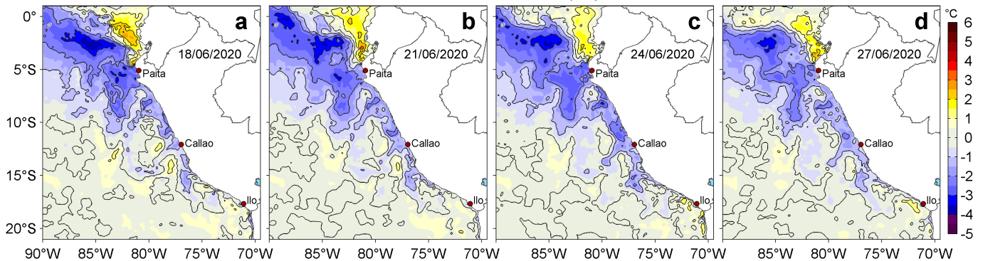
Figura 3. Anomalías de la temperatura superficial del mar (TSM, °C) para los días: a) 18, b) 21, c) 24 y d) 27 de junio de 2020. Las anomalías se calcularon respecto de la climatología para el periodo 2007-2016. Datos: OSTIA-UKMO-L4-GLOB-v2.0 (UK Met Office, 2012; Donlon et al, 2012). Procesamiento: LHF/AFIOF/DGIOCC/IMARPE.
