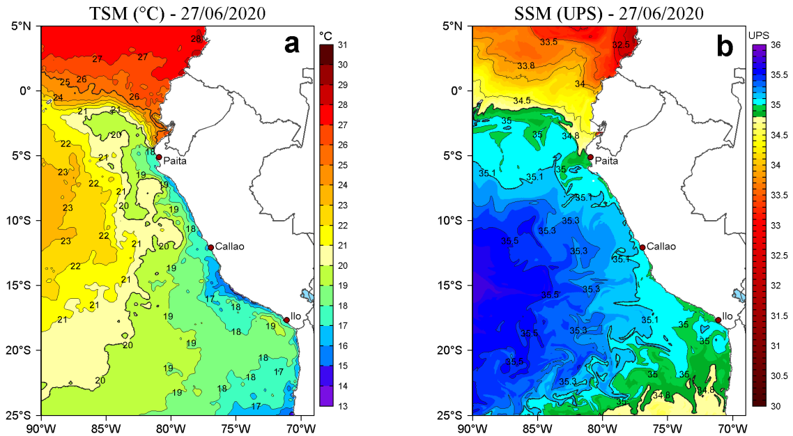
Figura 2. a) Temperatura superficial del mar (TSM, °C) y b) Salinidad superficial del mar (SSM, UPS), para el 27 de junio de 2020. Datos: OSTIA-UKMO-L4-GLOB-v2.0 (UK Met Office, 2012; Donlon et al, 2012) disponible en https://podaac.jpl.nasa.gov/dataset/OSTIA-UKMO-L4-GLOB-v2.0 para (a) y Hybrid Coordinate Ocean Model v. GOF3 3.1 (HYCOM; Halliwell et al., 1998; 2000; Bleck, 2001) para (b). Procesamiento: LHF/AFIOF/DGIOCC/IMARPE.
