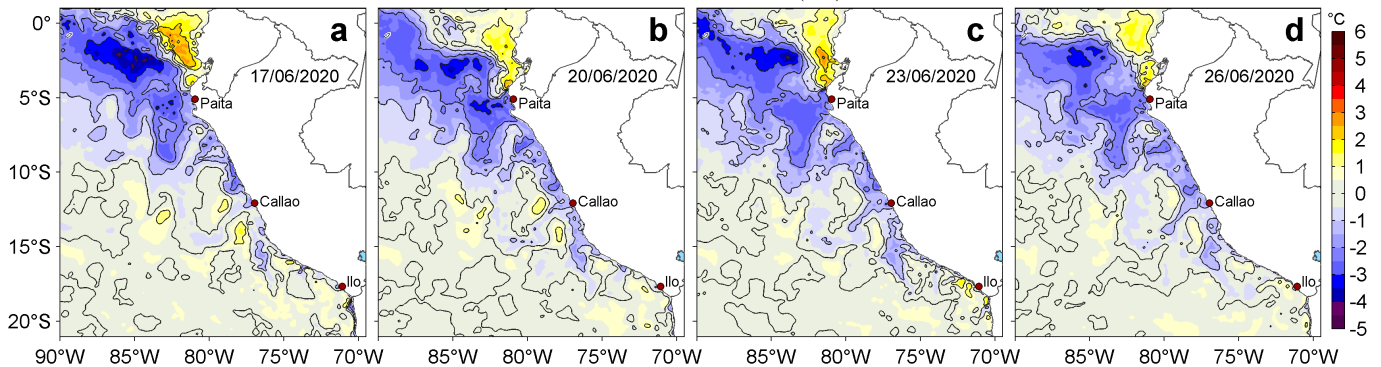
Figura 3. Anomalías de la temperatura superficial del mar (TSM, °C) para los días: a) 17, b) 20, c) 23 y d) 26 de junio de 2020. Las anomalías se calcularon respecto de la climatología para el periodo 2007-2016. Datos: OSTIA-UKMO-L4-GLOB-v2.0 (UK Met Office, 2012; Donlon et al, 2012). Procesamiento: LHF/AFIOF/DGIOCC/IMARPE.
