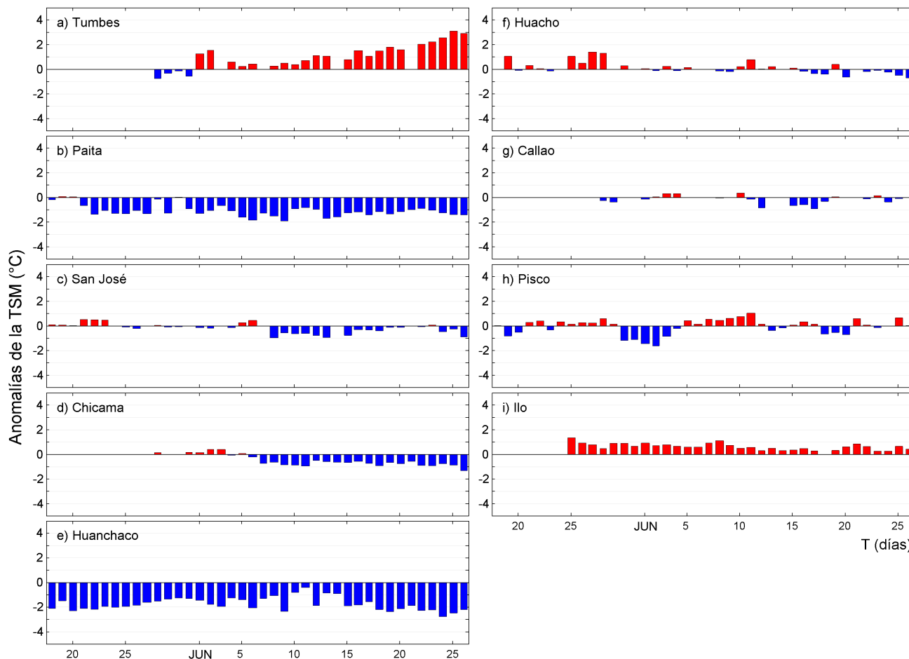
Figura 5. Variación del promedio diario de las anomalías de la temperatura superficial del mar (TSM, °C) en la red de estaciones costeras que administra IMARPE en el litoral peruano durante los últimos 40 días. Las anomalías se calcularon respecto del promedio climatológico pentadal (5 días) para el periodo que se indica en la Tabla 1. Datos y procesamiento: LHFM/AFIOF/DGIOCC/IMARPE.
