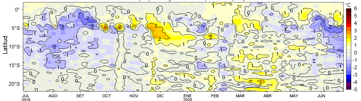
Figura 4. Variación promedio de las anomalías de la temperatura superficial del mar (TSM, °C) para una franja de 60 mn (~111 km) adyacente al litoral peruano para los últimos doce meses al 26 de junio de 2020. Datos: OSTIA-UKMO-L4-GLOB-v2.0 (UK Met. Office, 2012; Donlon et al, 2012) disponible en https://podaac.jpl.nasa.gov/dataset/OSTIA-UKMO-L4-GLOB-v2.0 . Las anomalías se calcularon con respecto al periodo 2007-2016. Procesamiento: LHF/AFIOF/DGIOCC/IMARPE.
