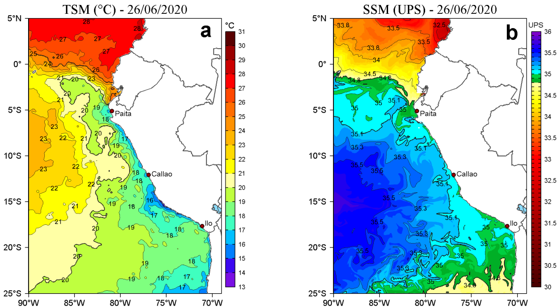
Figura 2. a) Temperatura superficial del mar (TSM, °C) y b) Salinidad superficial del mar (SSM, UPS), para el 26 de junio de 2020. Datos: OSTIA-UKMO-L4-GLOB-v2.0 (UK Met Office, 2012; Donlon et al, 2012) disponible en https://podaac.jpl.nasa.gov/dataset/OSTIA-UKMO-L4-GLOB-v2.0 para (a) y Hybrid Coordinate Ocean Model v. GOF3 3.1 (HYCOM; Halliwell et al., 1998; 2000; Bleck, 2001) para (b). Procesamiento: LHF/AFIOF/DGIOCC/IMARPE.
