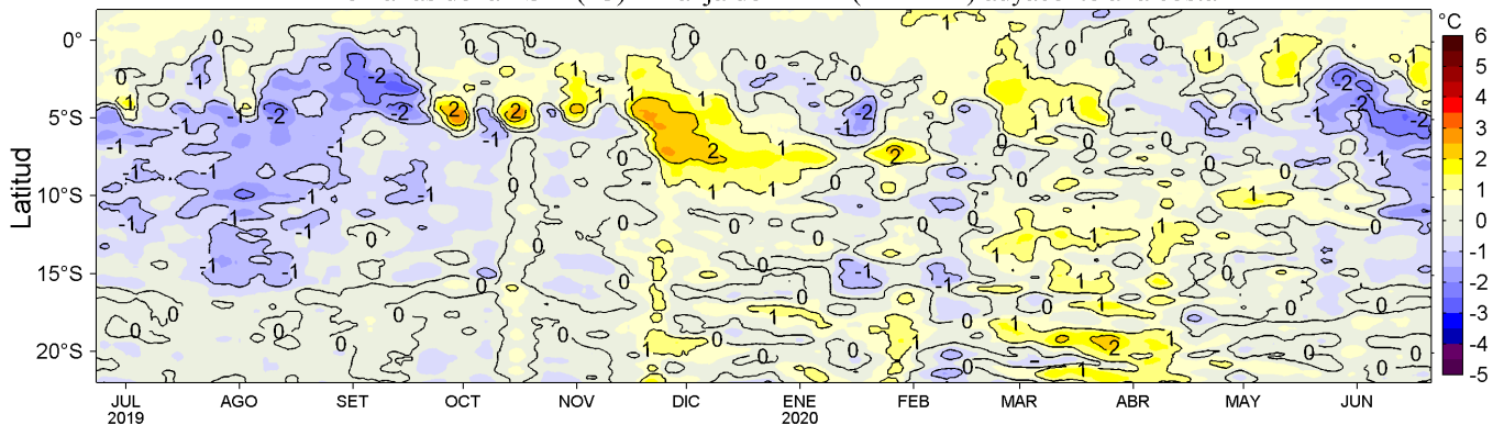
Figura 4. Variación promedio de las anomalías de la temperatura superficial del mar (TSM, °C) para una franja de 60 mn (~111 km) adyacente al litoral peruano para los últimos doce meses al 21 de junio de 2020. Datos: OSTIA-UKMO-L4-GLOB-v2.0 (UK Met. Office, 2012; Donlon et al, 2012) disponible en https://podaac.jpl.nasa.gov/dataset/OSTIA-UKMO-L4-GLOB-v2.0 . Las anomalías se calcularon con respecto al periodo 2007-2016. Procesamiento: LHFM/AFIOF/DGIOCC/IMARPE.
