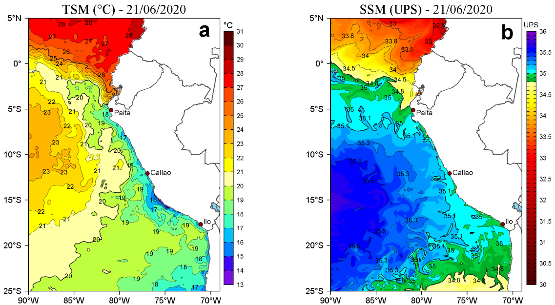
Figura 2. a) Temperatura superficial del mar (TSM, °C) y b) Salinidad superficial del mar (SSM, UPS), para el 21 de junio de 2020. Datos: OSTIA-UKMO-L4-GLOB-v2.0 (UK Met Office, 2012; Donlon et al, 2012) disponible en https://podaac.jpl.nasa.gov/dataset/OSTIA-UKMO-L4-GLOB-v2.0 para (a) y Hybrid Coordinate Ocean Model v. GOFS 3.1 (HYCOM; Halliwell et al., 1998; 2000; Bleck, 2001) para (b). Procesamiento: LHFM/AFIOF/DGIOCC/IMARPE.
