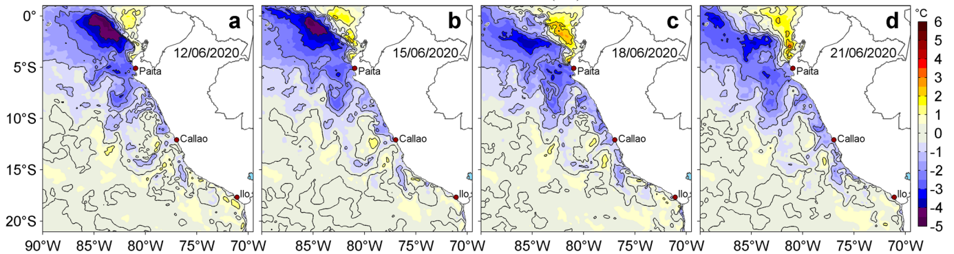
Figura 3. Anomalías de la temperatura superficial del mar (TSM, °C) para los días: a) 12, b) 15, c) 18 y d) 21 de junio de 2020. Las anomalías se calcularon respecto de la climatología para el periodo 2007-2016. Datos: OSTIA-UKMO-L4-GLOB-v2.0 (UK Met Office, 2012; Donlon et al, 2012). Procesamiento: LHFM/AFIOF/DGIOCC/IMARPE.
