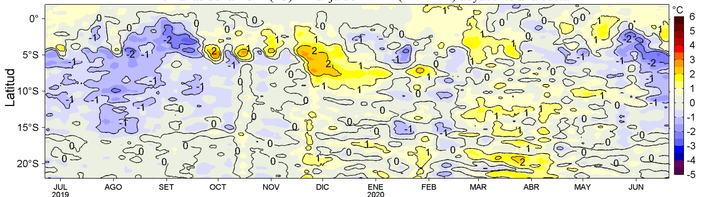
Figura 4. Variación promedio de las anomalías de la temperatura superficial del mar (TSM, °C) para una franja de 60 mn (~111 km) adyacente al litoral peruano para los últimos doce meses al 20 de junio de 2020. Datos: OSTIA-UKMO-L4-GLOB-v2.0 (UK Met. Office, 2012; Donlon et al, 2012) disponible en https://podaac.jpl.nasa.gov/dataset/OSTIA-UKMO-L4-GLOB-v2.0 . Las anomalías se calcularon con respecto al periodo 2007-2016. Procesamiento: LHFm/AFIOF/DGIOCC/IMARPE.
