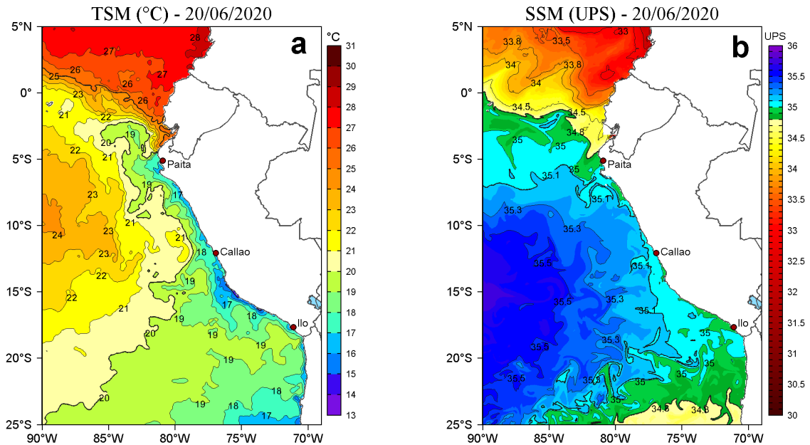
Figura 2. a) Temperatura superficial del mar (TSM, °C) y b) Salinidad superficial del mar (SSM, UPS), para el 20 de junio de 2020. Datos: OSTIA-UKMO-L4-GLOB-v2.0 (UK Met Office, 2012; Donlon et al, 2012) disponible en https://podaac.jpl.nasa.gov/dataset/OSTIA-UKMO-L4-GLOB-v2.0 para (a) y Hybrid Coordinate Ocean Model v. GOFS 3.1 (HYCOM; Halliwell et al., 1998; 2000; Bleck, 2001) para (b). Procesamiento: LHFm/AFIOF/DGIOCC/IMARPE.
