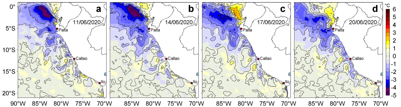
Figura 3. Anomalías de la temperatura superficial del mar (TSM, °C) para los días: a) 11, b) 14, c) 17 y d) 20 de junio de 2020. Las anomalías se calcularon respecto de la climatología para el periodo 2007-2016. Datos: OSTIA-UKMO-L4-GLOB-v2.0 (UK Met Office, 2012; Donlon et al, 2012). Procesamiento: LHFm/AFIOF/DGIOCC/IMARPE.
