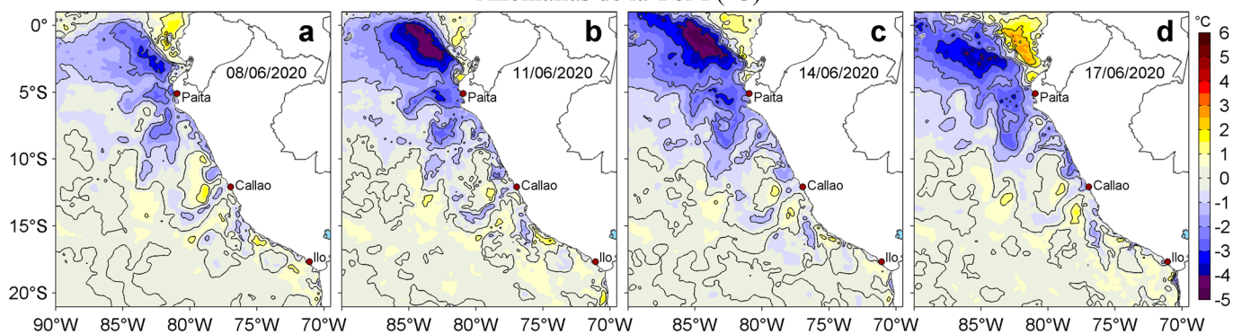
Figura 3. Anomalías de la temperatura superficial del mar (TSM, °C) para los días: a) 08, b) 11, c) 14 y d) 17 de junio de 2020. Las anomalías se calcularon respecto de la climatología para el periodo 2007-2016. Datos: OSTIA-UKMO-L4-GLOB-v2.0 (UK Met Office, 2012; Donlon et al, 2012). Procesamiento: LHFM/AFIOF/DGIOCC/IMARPE.
