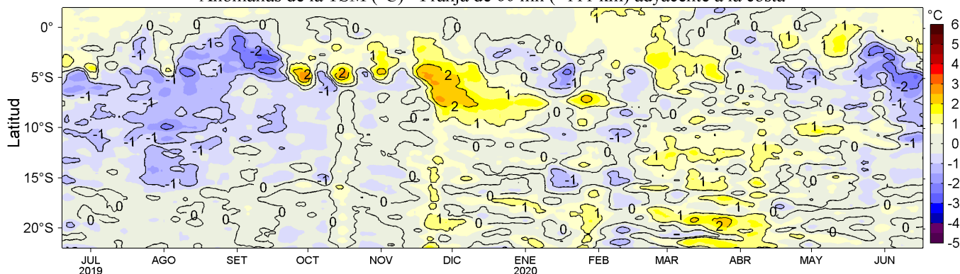
Figura 4. Variación promedio de las anomalías de la temperatura superficial del mar (TSM, °C) para una franja de 60 mn (~111 km) adyacente al litoral peruano para los últimos doce meses al 17 de junio de 2020. Datos: OSTIA-UKMO-L4-GLOB-v2.0 (UK Met. Office, 2012; Donlon et al, 2012) disponible en https://podaac.jpl.nasa.gov/dataset/OSTIA-UKMO-L4-GLOB-v2.0 . Las anomalías se calcularon con respecto al periodo 2007-2016. Procesamiento: LHFM/AFIOF/DGIOCC/IMARPE.
