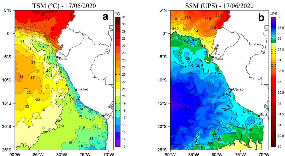
Figura 2. a) Temperatura superficial del mar (TSM, °C) y b) Salinidad superficial del mar (SSM, UPS), para el 17 de junio de 2020. Datos: OSTIA-UKMO-L4-GLOB-v2.0 (UK Met Office, 2012; Donlon et al, 2012) disponible en https://podaac.jpl.nasa.gov/dataset/OSTIA-UKMO-L4-GLOB-v2.0 para (a) y Hybrid Coordinate Ocean Model v. GOFS 3.1 (HYCOM; Halliwell et al., 1998; 2000; Bleck, 2001) para (b). Procesamiento: LHFM/AFIOF/DGIOCC/IMARPE.
