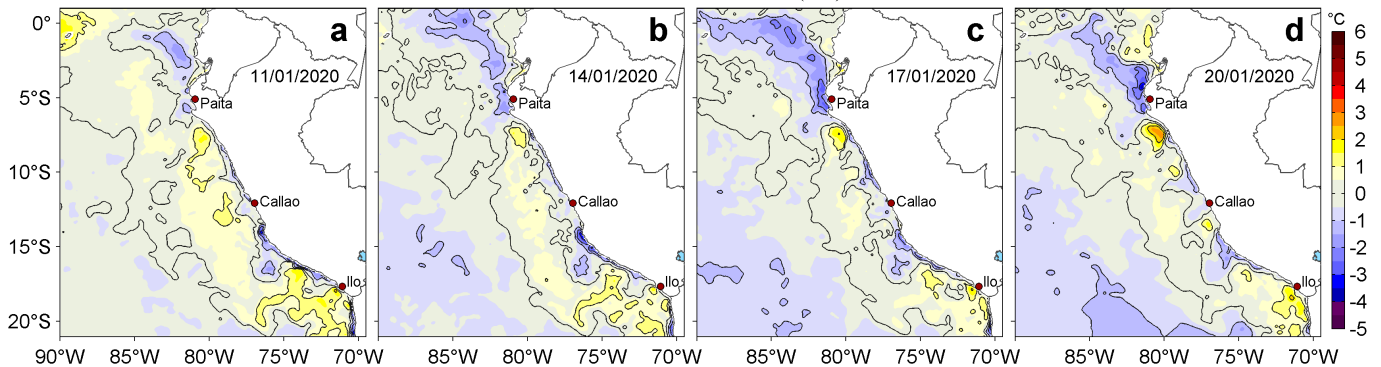
Figura 3. Anomalías de la temperatura superficial del mar (TSM, °C) para los días: a) 11, b) 14, c) 17 y d) 20 de enero de 2020. Las anomalías se calcularon respecto de la climatología para el periodo 2007-2016. Datos: OSTIA-UKMO-L4-GLOB-v2.0 (UK Met Office, 2012; Donlon et al, 2012). Procesamiento: LHF/AFIOF/DGIOCC/IMARPE.
