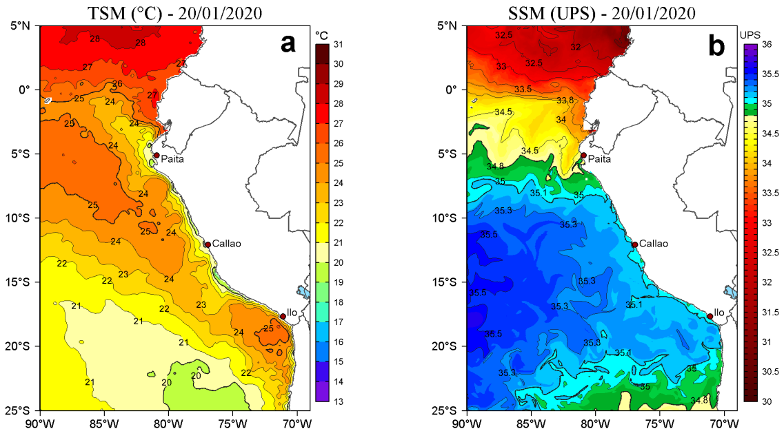
Figura 2. a) Temperatura superficial del mar (TSM, °C) y b) Salinidad superficial del mar (SSM, UPS), para el 20 de enero de 2020. Datos: OSTIA-UKMO-L4-GLOB-v2.0 (UK Met Office, 2012; Donlon et al, 2012) disponible en https://podaac.jpl.nasa.gov/dataset/OSTIA-UKMO-L4-GLOB-v2.0 para (a) y Hybrid Coordinate Ocean Model v. GOF3 3.1 (HYCOM; Halliwell et al., 1998; 2000; Bleck, 2001) para (b). Procesamiento: LHF/AFIOF/DGIOCC/IMARPE.
