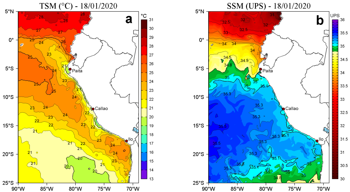
Figura 2. a) Temperatura superficial del mar (TSM, °C) y b) Salinidad superficial del mar (SSM, UPS), para el 18 de enero de 2020. Datos: OSTIA-UKMO-L4-GLOB-v2.0 (UK Met Office, 2012; Donlon et al, 2012) disponible en https://podaac.jpl.nasa.gov/dataset/OSTIA-UKMO-L4-GLOB-v2.0 para (a) y Hybrid Coordinate Ocean Model v. GOF3 3.1 (HYCOM; Halliwell et al., 1998; 2000; Bleck, 2001) para (b). Procesamiento: LHFM/AFIOF/DGIOCC/IMARPE.
