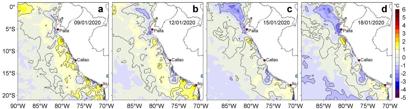
Figura 3. Anomalías de la temperatura superficial del mar (TSM, °C) para los días: a) 09, b) 12, c) 15 y d) 18 de enero de 2020. Las anomalías se calcularon respecto de la climatología para el periodo 2007-2016. Datos: OSTIA-UKMO-L4-GLOB-v2.0 (UK Met Office, 2012; Donlon et al, 2012). Procesamiento: LHFM/AFIOF/DGIOCC/IMARPE.
