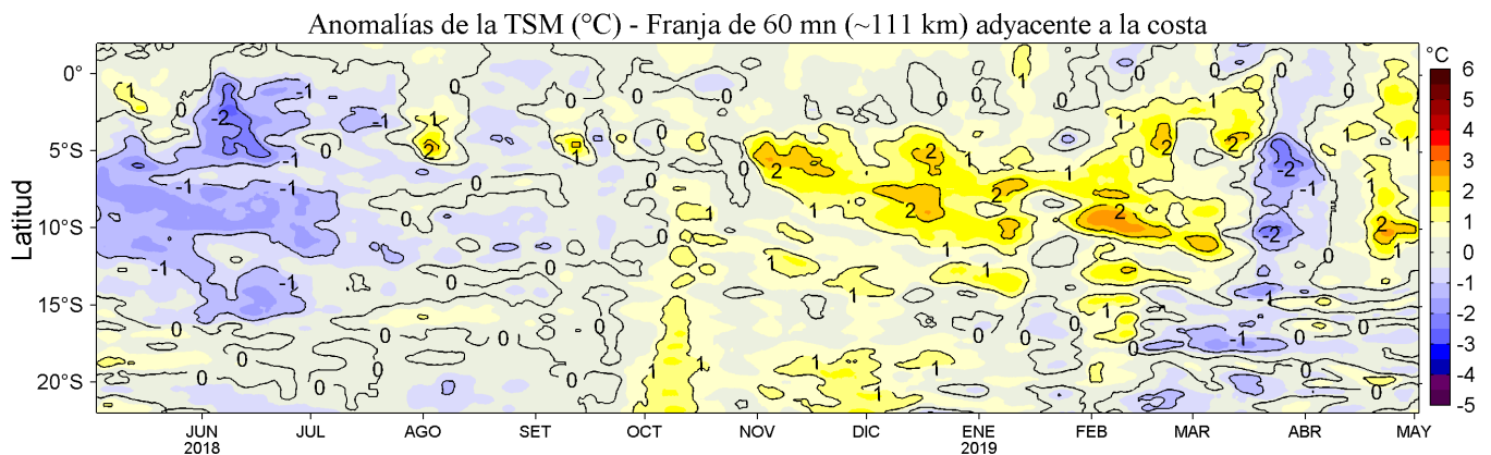
Figura 4. Variación promedio de las anomalías de la temperatura superficial del mar (TSM, °C) para una franja de 60 mn (~111 km) adyacente al litoral peruano para los últimos doce meses al 02 de mayo de 2019. Datos: OSTIA-UKMO-L4-GLOB-v2.0 (UK Met. Office, 2012; Donlon et al, 2012) disponible en https://podaac.jpl.nasa.gov/dataset/OSTIA-UKMO-L4-GLOB-v2.0 . Las anomalías se calcularon con respecto al periodo 2007-2016. Procesamiento: LHF/AFIOF/DGIOCC/IMARPE.
