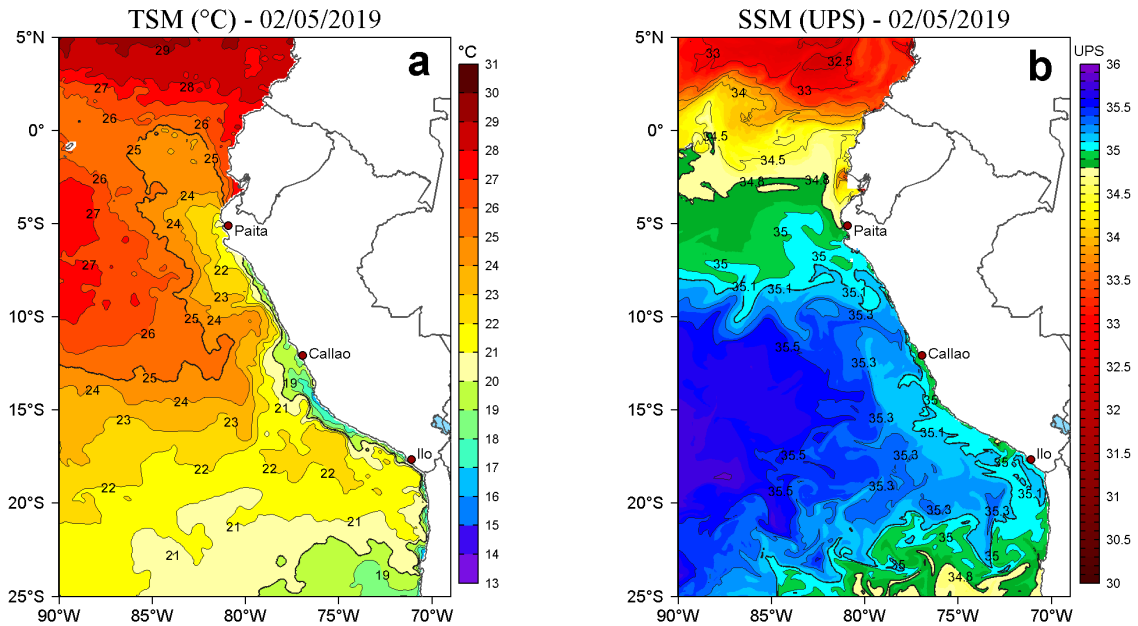
Figura 2. a) Temperatura superficial del mar (TSM, °C) y b) Salinidad superficial del mar (SSM, UPS), para el 02 de mayo de 2019. Datos: OSTIA-UKMO-L4-GLOB-v2.0 (UK Met Office, 2012; Donlon et al, 2012) disponible en https://podaac.jpl.nasa.gov/dataset/OSTIA-UKMO-L4-GLOB-v2.0 para (a) y Hybrid Coordinate Ocean Model v. GOF3 3.1 (HYCOM; Halliwell et al., 1998; 2000; Bleck, 2001) para (b). Procesamiento: LHF/AFIOF/DGIOCC/IMARPE.
