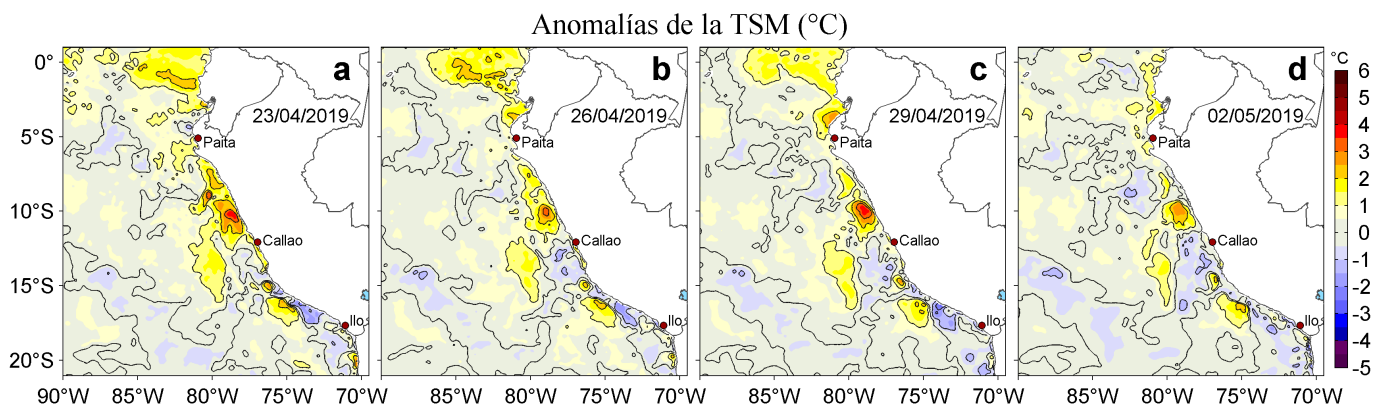
Figura 3. Anomalías de la temperatura superficial del mar (TSM, °C) para los días: a) 23, b) 26 y c) 29 de abril y d) 02 de mayo de 2019. Las anomalías se calcularon respecto de la climatología para el periodo 2007-2016. Datos: OSTIA-UKMO-L4-GLOB-v2.0 (UK Met Office, 2012; Donlon et al, 2012). Procesamiento: LHF/AFIOF/DGIOCC/IMARPE.
