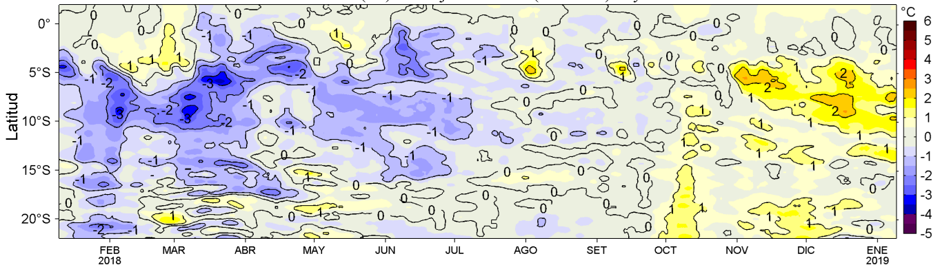
Figura 4. Variación promedio de las anomalías de la temperatura superficial del mar (TSM, °C) para una franja de 60 mn (~111 km) adyacente al litoral peruano para los últimos doce meses al 09 de enero de 2019. Datos: OSTIA-UKMO-L4-GLOB-v2.0 (UK Met. Office, 2012; Donlon et al, 2012) disponible en https://podaac.jpl.nasa.gov/dataset/OSTIA-UKMO-L4-GLOB-v2.0 . Las anomalías se calcularon con respecto al periodo 2007-2016. Procesamiento: LHF/AFIOF/DGIOCC/IMARPE.
