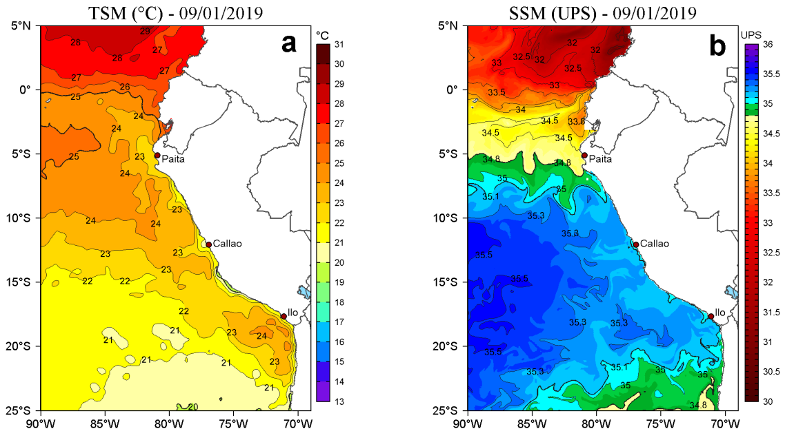
Figura 2. a) Temperatura superficial del mar (TSM, °C) y b) Salinidad superficial del mar (SSM, UPS) para el 09 de enero de 2019. Datos: OSTIA-UKMO-L4-GLOB-v2.0 (UK Met Office, 2012; Donlon et al, 2012) disponible en https://podaac.jpl.nasa.gov/dataset/OSTIA-UKMO-L4-GLOB-v2.0 para (a) y Hybrid Coordinate Ocean Model v. GOF3 3.1 (HYCOM; Halliwell et al., 1998; 2000; Bleck, 2001) para (b). Procesamiento: LHF/AFIOF/DGIOCC/IMARPE.
