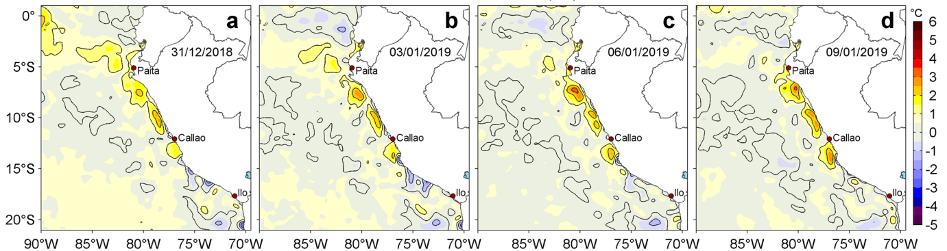
Figura 3. Anomalías de la temperatura superficial del mar (TSM, °C) para los días: a) 31 de diciembre del 2018, b) 03, c) 06 y d) 09 de enero de 2019. Las anomalías se calcularon respecto de la climatología para el periodo 2007-2016. Datos: OSTIA-UKMO-L4-GLOB-v2.0 (UK Met Office, 2012; Donlon et al, 2012). Procesamiento: LHF/AFIOF/DGIOCC/IMARPE.
