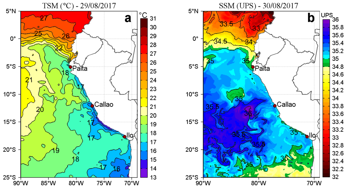
Figura 2. a) Temperatura superficial del mar (°C) y b) Salinidad superficial del mar (UPS) para el 29 y 30 de agosto respectivamente. Datos: OSTIA-UKMO-L4-GLOB-v2.0 (UK Met Office, 2012; Donlon et al, 2012) disponible en https://podaac.jpl.nasa.gov/dataset/OSTIA-UKMO-L4-GLOB-v2.0 para (a) y Hybrid Coordinate Ocean Model (HYCOM; Halliwell et al., 1998; 2000; Bleck, 2001) para (b). Procesamiento: LHF/AFIOF/DGIOCC/IMARPE.
