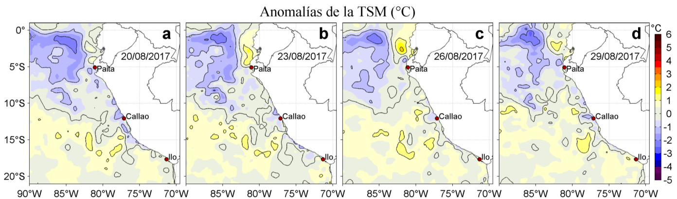
Figura 3. Anomalías de la Temperatura Superficial del Mar (°C) para los días: a) 20, b) 23, c) 26, y d) 29 de agosto de 2017. Las anomalías se calcularon respecto de la climatología para el periodo 2007-2016. Datos: OSTIA-UKMO-L4-GLOB-v2.0 (UK Met Office, 2012; Donlon et al, 2012). Procesamiento: LHF/AFIOF/DGIOCC/IMARPE.
