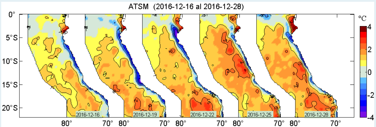
Figura 2. Anomalías de la temperatura superficial del agua (°C) en el mar peruano, cada tres días, entre el 16 y 28 de diciembre del 2016. Datos: AVHRR Global Reyn_SmithOiv2R (Reynolds, et. al., 2007) de CMB/EMC/NCEP de la NOAA. Procesamiento: IMARPE.
