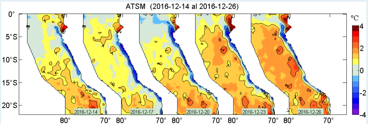
Figura 2. Anomalías de la temperatura superficial del agua (°C) en el mar peruano, cada tres días, entre el 14 y 26 de diciembre del 2016. Datos: AVHRR Global Reyn_SmithOiv2R (Reynolds, et. al., 2007) de CMB/EMC/NCEP de la NOAA. Procesamiento: IMARPE.
