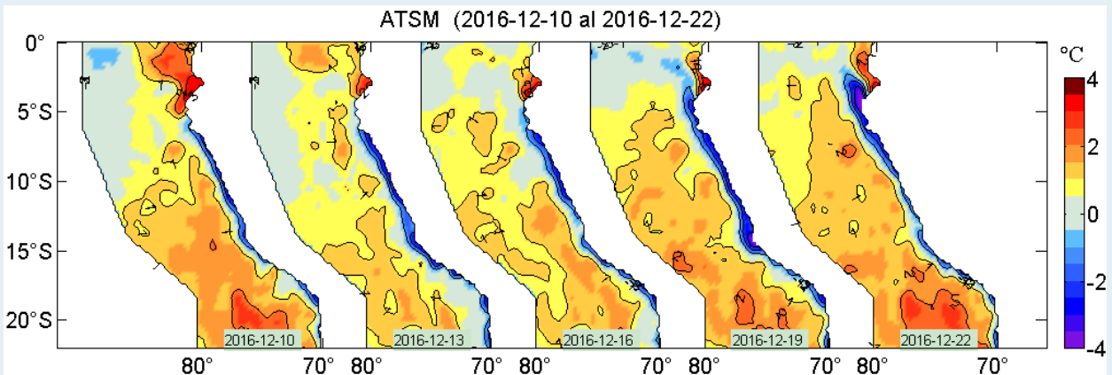
Figura 2. Anomalías de la temperatura superficial del agua (°C) en el mar peruano, cada tres días, entre el 10 y 22 de diciembre del 2016. Datos: AVHRR Global Reyn_SmithOiv2R (Reynolds, et. al., 2007) de CMB/EMC/NCEP de la NOAA. Procesamiento: IMARPE.
