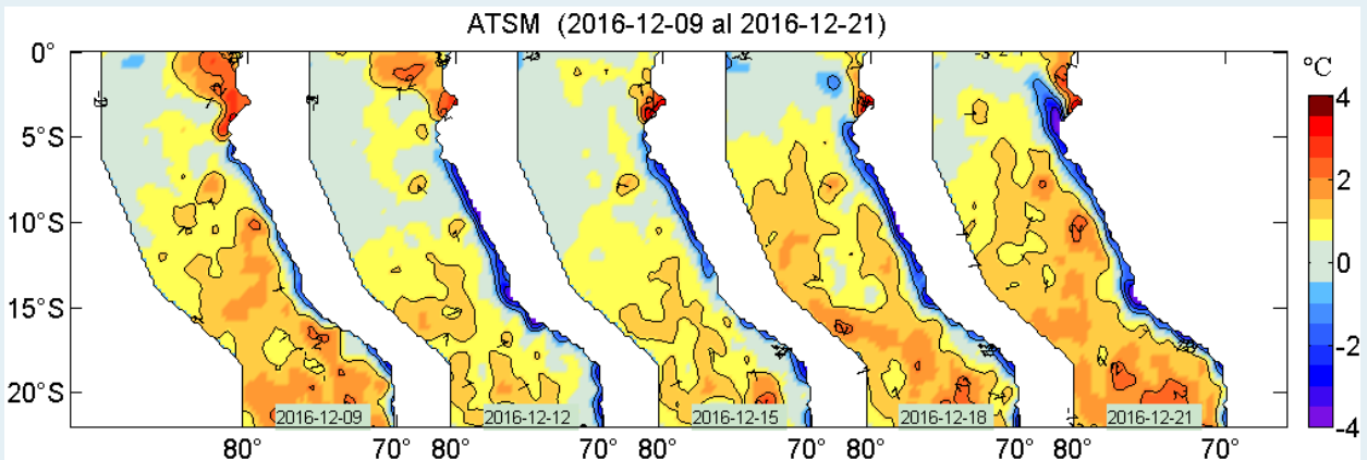
Figura 2. Anomalías de la temperatura superficial del agua (°C) en el mar peruano, cada tres días, entre el 09 y 21 de diciembre del 2016. Datos: AVHRR Global Reyn_SmithOiv2R (Reynolds, et. al., 2007) de CMB/EMC/NCEP de la NOAA. Procesamiento: IMARPE.
