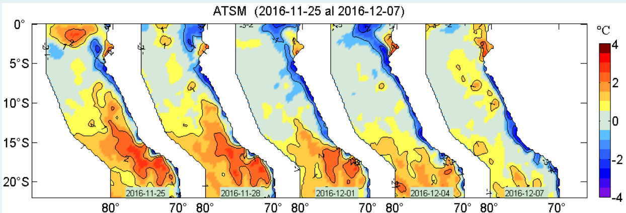
Figura 2. Anomalías de la temperatura superficial del agua (°C) en el mar peruano, cada tres días, entre el 25 de noviembre y 07 de diciembre del 2016. Datos: AVHRR Global Reyn_SmithOiv2R (Reynolds, et. al., 2007) de CMB/EMC/NCEP de la NOAA. Procesamiento: IMARPE.
