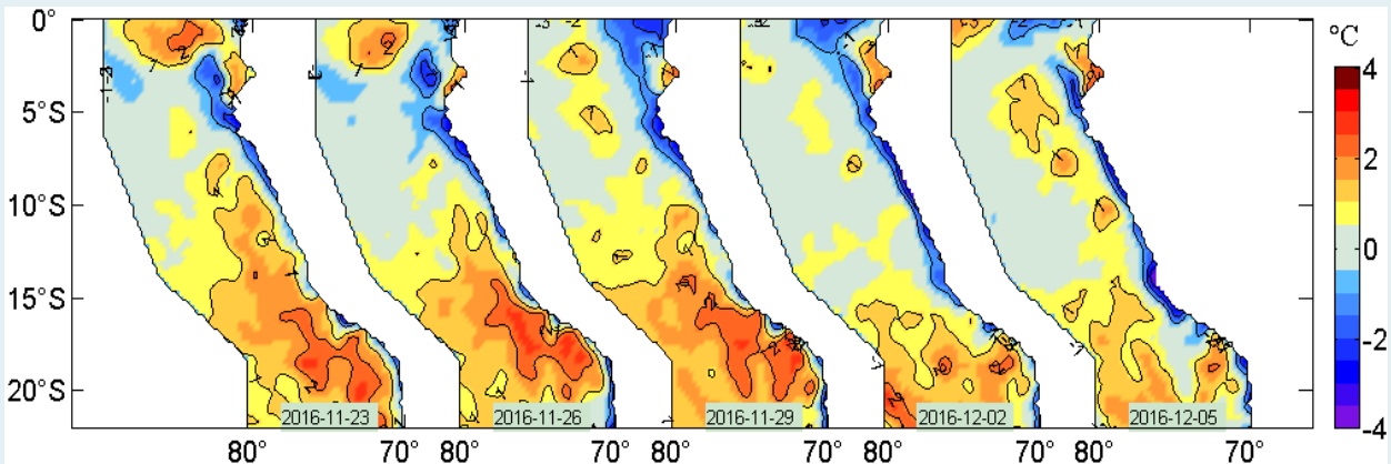
Figura 2. Anomalías de la temperatura superficial del agua (°C) en el mar peruano, cada tres días, entre el 23 de noviembre y 05 de diciembre del 2016. Datos: AVHRR Global Reyn_SmithOiv2R (Reynolds, et. al., 2007) de CMB/EMC/NCEP de la NOAA. Procesamiento: IMARPE.
