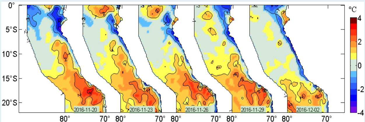
Figura 2. Anomalías de la temperatura superficial del agua (°C) en el mar peruano, cada tres días, entre el 20 de noviembre y 02 de diciembre del 2016. Datos: AVHRR Global Reyn_SmithOiv2R (Reynolds, et. al., 2007) de CMB/EMC/NCEP de la NOAA. Procesamiento: IMARPE.
