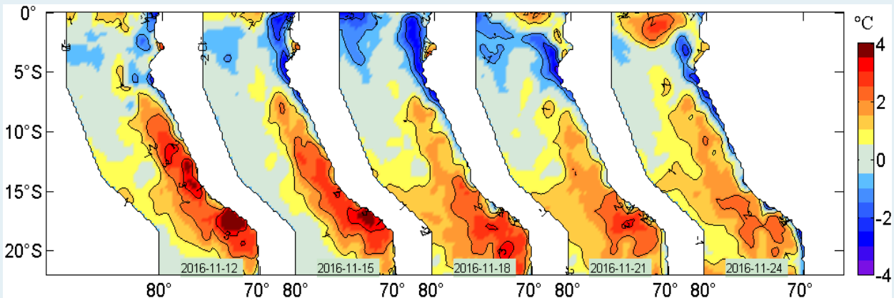
Figura 2. Anomalías de la temperatura superficial del agua (°C) en el mar peruano, cada tres días, entre el 12 y 24 de noviembre del 2016. Datos: AVHRR Global Reyn_SmithOiv2R (Reynolds, et. al., 2007) de CMB/EMC/NCEP de la NOAA. Procesamiento: IMARPE.
