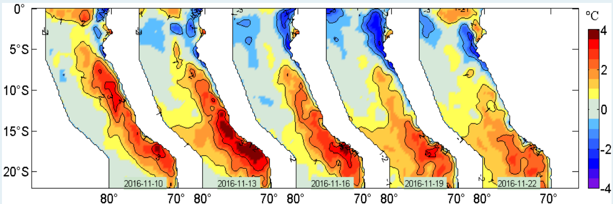
Figura 2. Anomalías de la temperatura superficial del agua (°C) en el mar peruano, cada tres días, entre el 10 y 22 de noviembre del 2016. Datos: AVHRR Global Reyn_SmithOiv2R (Reynolds, et. al., 2007) de CMB/EMC/NCEP de la NOAA. Procesamiento: IMARPE.
