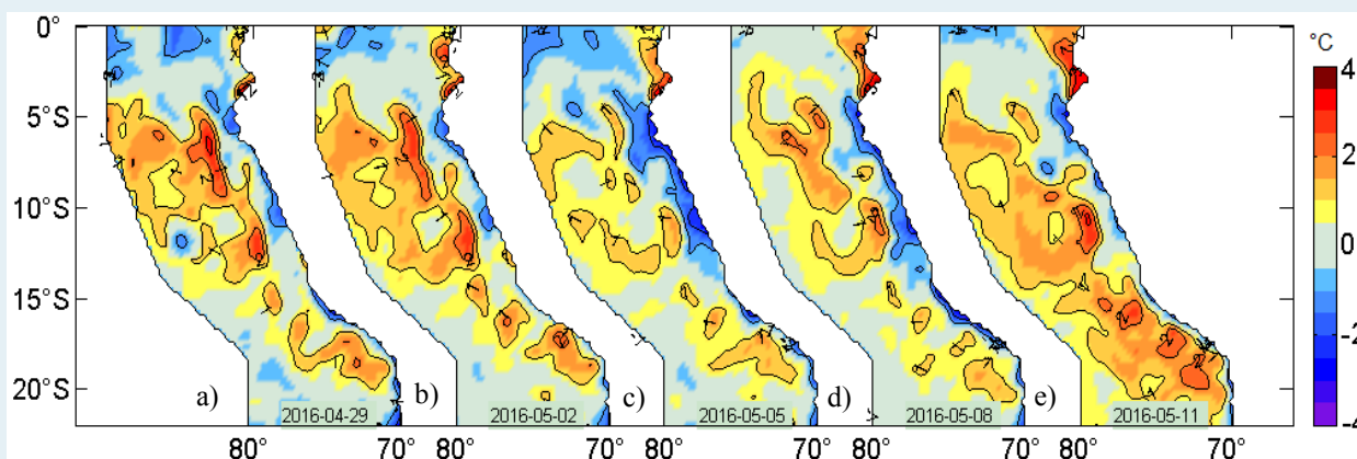
Figura 2. Anomalías de la temperatura superficial del agua (°C) en el mar peruano, cada tres días, entre el 29 de abril y 11 de mayo del 2016. Datos: AVHRR Global Reyn_SmithOiv2R (Reynolds, et. al., 2007) de CMB/EMC/NCEP de la NOAA. Procesamiento: IMARPE.
