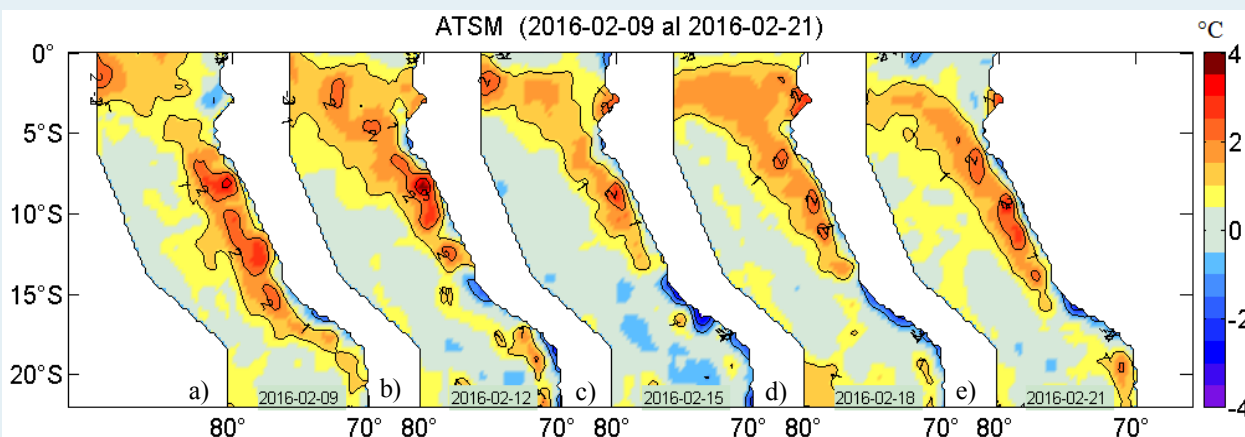
Figura 2. Anomalías de la temperatura superficial del agua (°C) en el mar peruano, cada tres días, entre el 09 y 21 de febrero del 2016. Datos: AVHRR de NOAA. Procesamiento: IMARPE.
