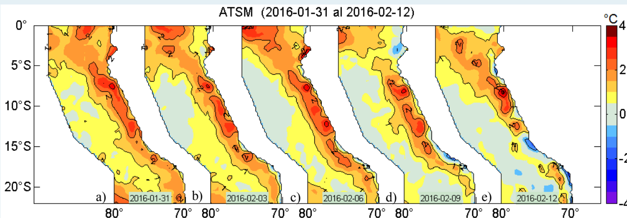
Figura 2. Anomalías de la temperatura superficial del agua (°C) en el mar peruano, cada tres días, entre el 31 de enero y 12 de febrero del 2016. Datos: AVHRR/NOAA. Procesamiento: IMARPE.
