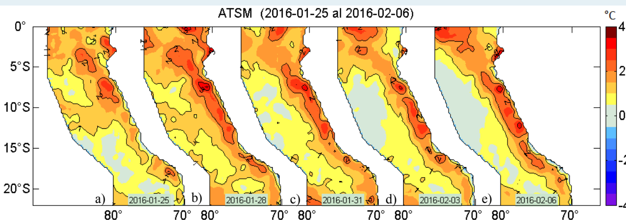
Figura 2. Anomalías de la temperatura superficial del agua (°C) en el mar peruano, cada tres días, entre el 25 de enero y 06 de febrero del 2016. Datos: AVHRR/NOAA. Procesamiento: IMARPE.
