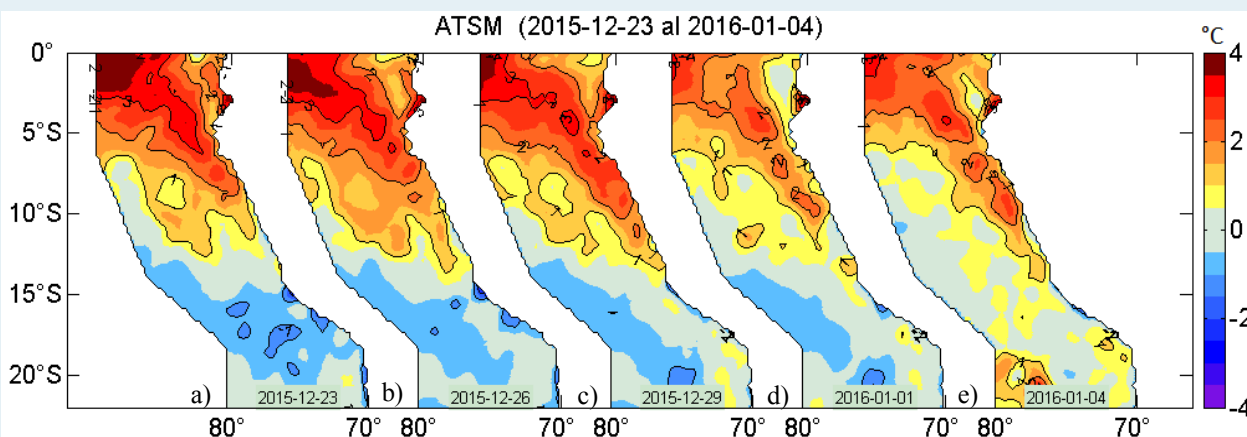
Figura 2. Anomalías de la temperatura superficial del agua (°C) en el mar peruano, cada tres días, entre el 23 de diciembre de 2015 al 4 de enero del 2016. Datos: AVHRR/NOAA. Procesamiento: IMARPE.
